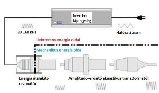
1. ábra. Az ultrahangos ponthegeztés sematikus ábrája [1]
