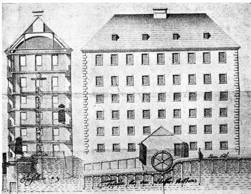
1. Az óbudai filatorium homlokzata és keresztmetszete.
