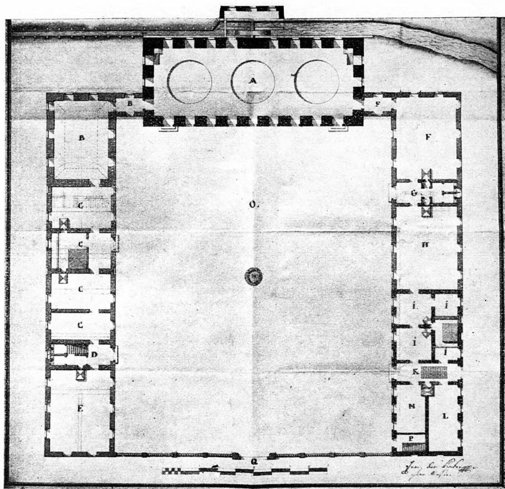
2. Az óbudai filatorium alaprajza.
