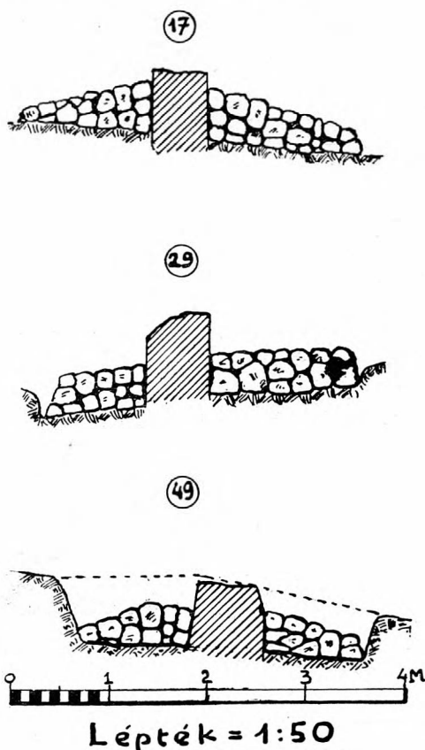
6. A vadaskert falának keresztmetszetei.
