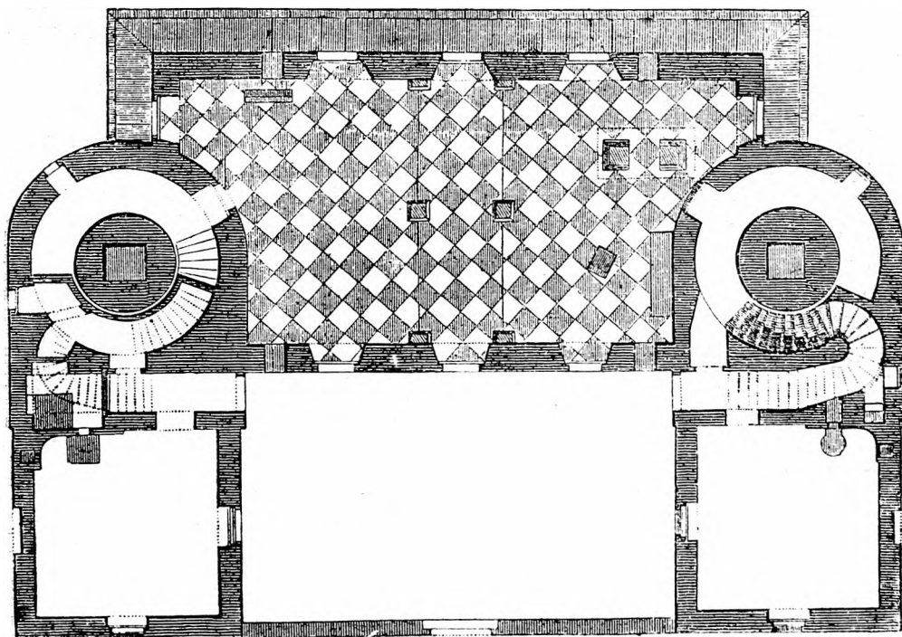
A gellérthegy csillagvizsgáló alaprajza.
