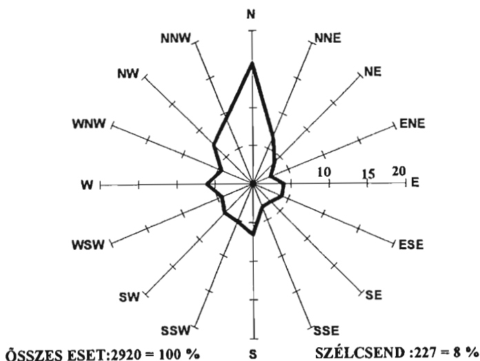
A szélirányok gyakorisága (%) – veszprémi főállomás, 1994
