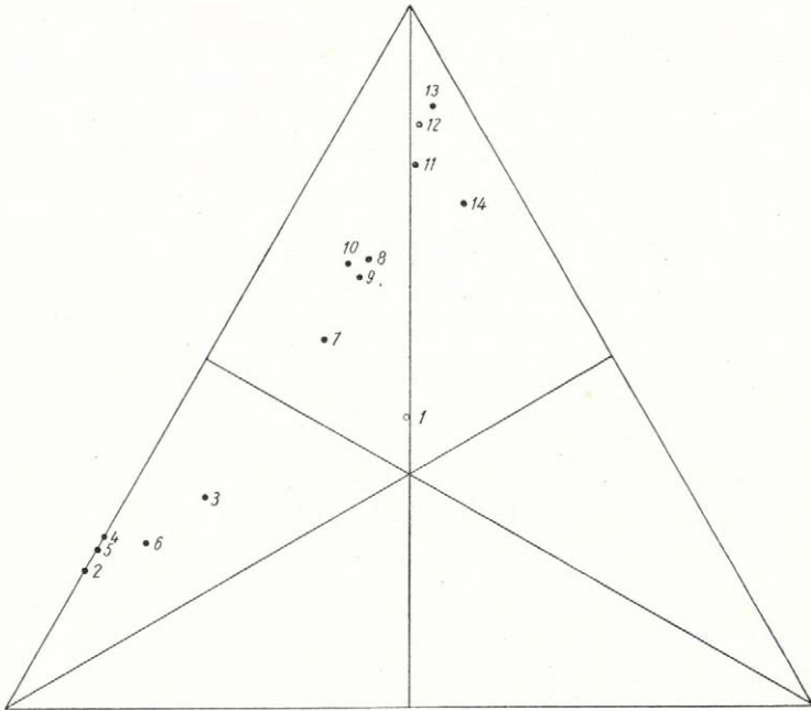
Die Projektionspunkte im OSANNSCHEN Dreieck.
