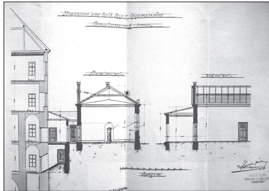
23. Tervrajz a tornaterem felépítésére a gimnázium épületéhez csatlatkoztatva, 1899 (nem valósult meg), metszetek. 65
