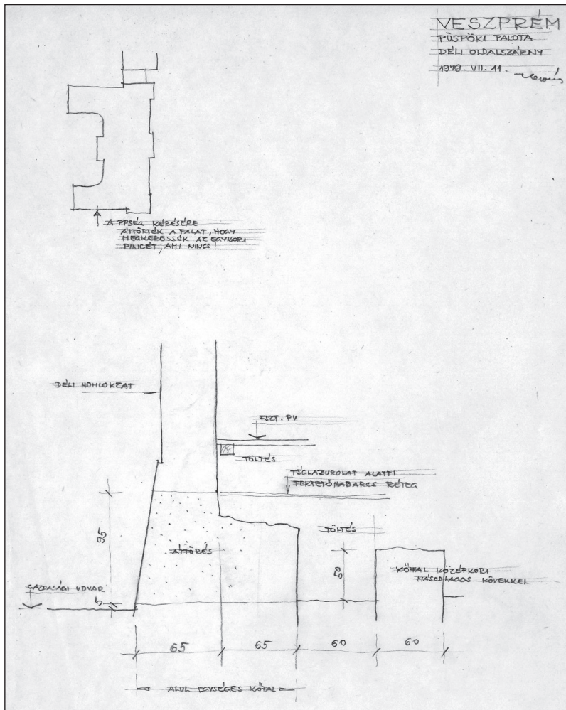
Metszet az áttörésekről (Rajz: Koppány Tibor)
