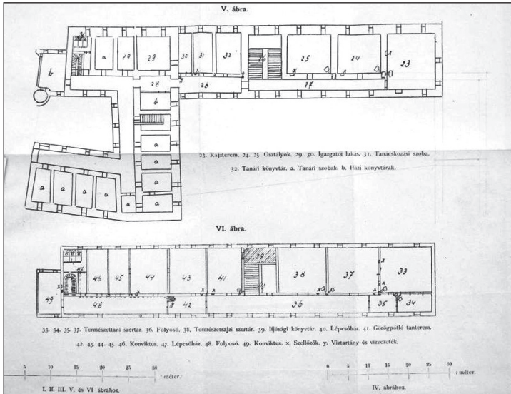
7. Az 1893-as átépítés utáni funkcionális elrendezést bemutató alaprajzai Bolgár Mihály tanulmányában. 50
