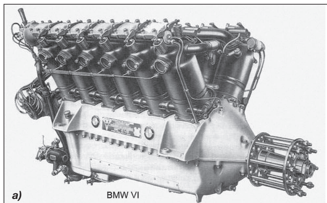
1. ábra. BMW VI. V12 repülőgépmotor a) és Mikulin M17 motor b). A két motor konstrukciós hasonlósága egyértelmű [16]
