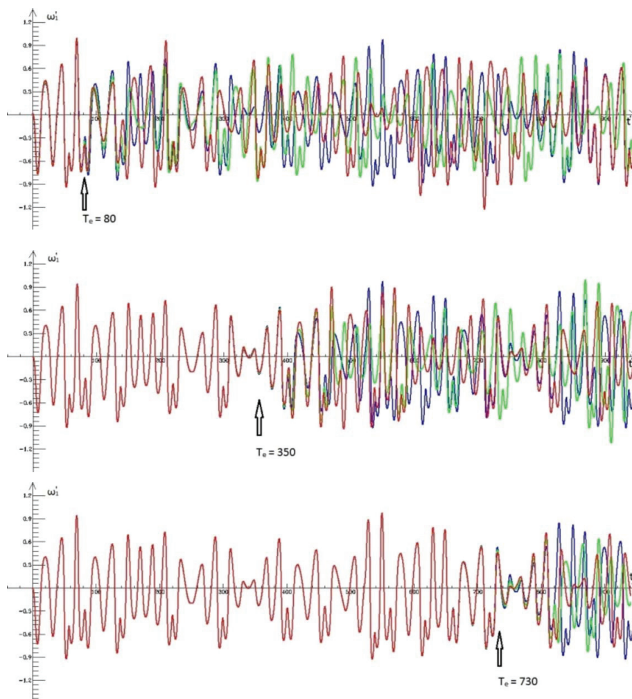
12. ábra. Néhány fáklyadiagram, rendre \Delta\omega'_{10} = 10^{-2} ; 10^{-6} és 10^{-10} kezdőérték-eltéréssel. A további közös értékek: D = 2,4 ; k = 0,02 ; \varphi_{10} = 0 ; \varphi_{20} = 0 ; T'_{20} = 20 ; \omega'_{10} = 0 + \Delta\omega'_{10} . (A Dynamic Solver program által szolgáltatott ábra.)
