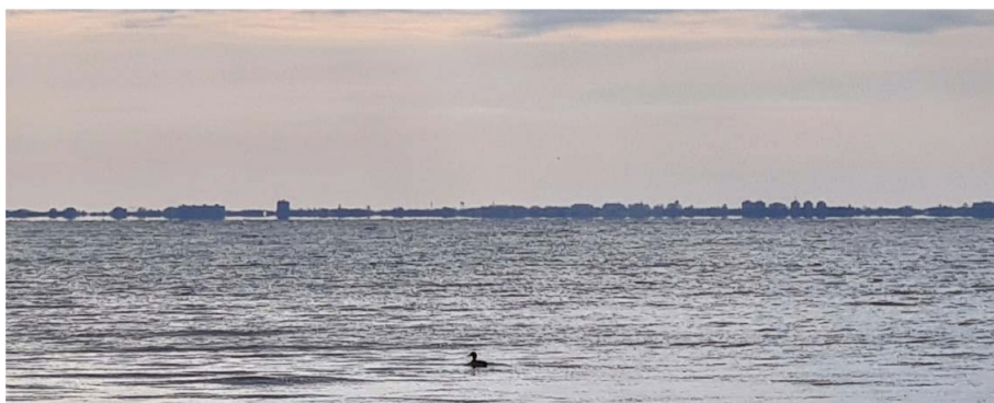
1. ábra. Délibáb a Balaton fölött (Siófok Balatonfüredről fotózva). Az épületek és fák a távolban „visszatükröződnek” egy vízszintes vonal mentén.
