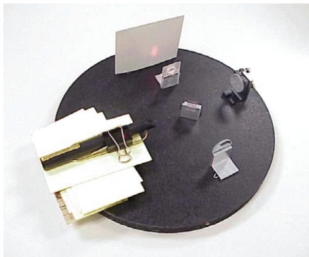
7. ábra. A diákok által összeállítható asztali interferométer [11].
