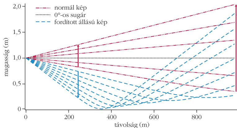
2. ábra. Fény elhajlása aszfaltút fölött. A környezeti hőmérséklet 38,5\text{ }^{\circ}\text{C} , a sugarak -0,18^{\circ} – 0,06^{\circ} alatt indulnak a vízszinteshez képest 0,02^{\circ} -os lépésekben.
