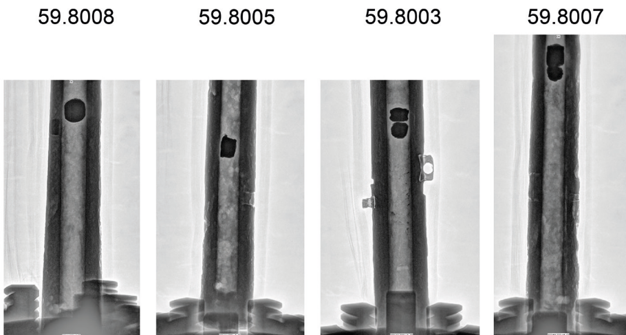
5. kép: A négy töltött cső röntgenképe
