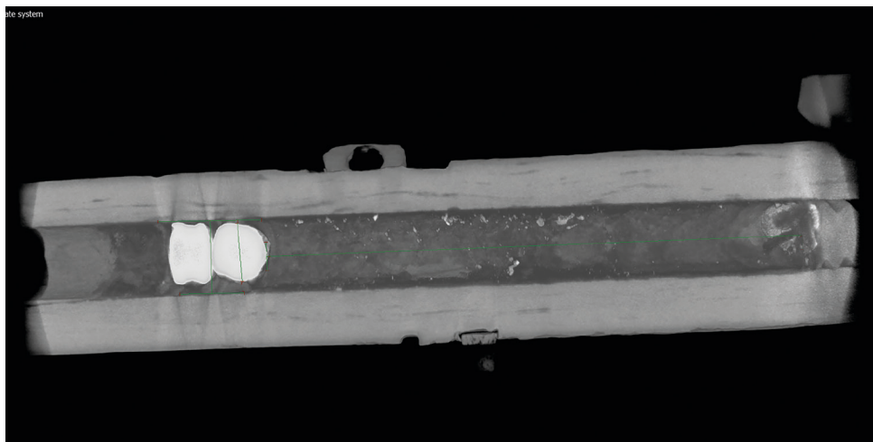
7. kép: A csőfar 3D modellje, jól láthatóak a csőfánál a löporszemcsék
