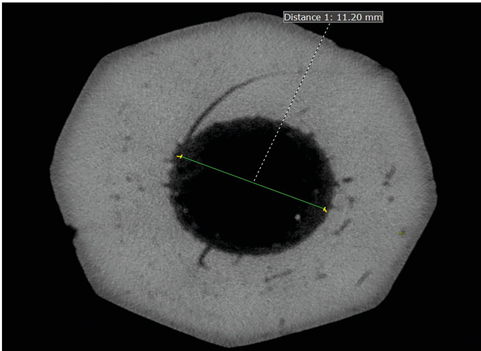
9. kép: A furatátmérő mérése a modellen. Jól látható a cső alapanyagának átlapolása
