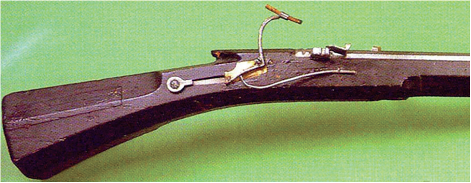
42. kép: A grazi Landeszeughausban őrzött első olyan ismert kézi lőfegyver, mely a későbbi muskéták jellemzőit mutatja (Ethnographic Arms & Armor)
