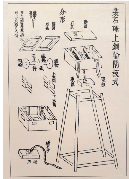
45. kép: A gyújtórendszer
