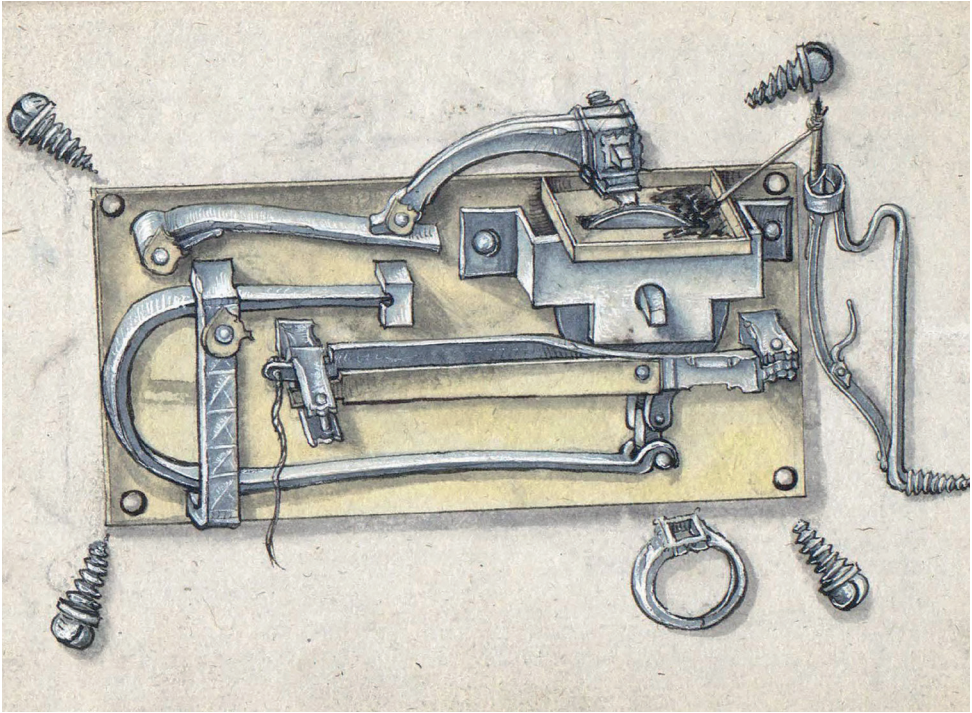
47. kép: Löffelholz rugós gyújtószerkezete
