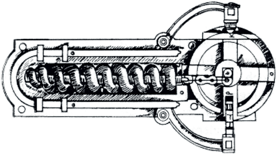
49. kép: Da Vinci spirálrugós lakatja
