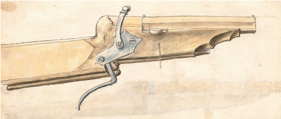
2. kép: Martin Merz könnyű puskája (arkebúz/pisztoly) kanócos lakatlemezzel, emelőkaros elsütőszerkezettel
