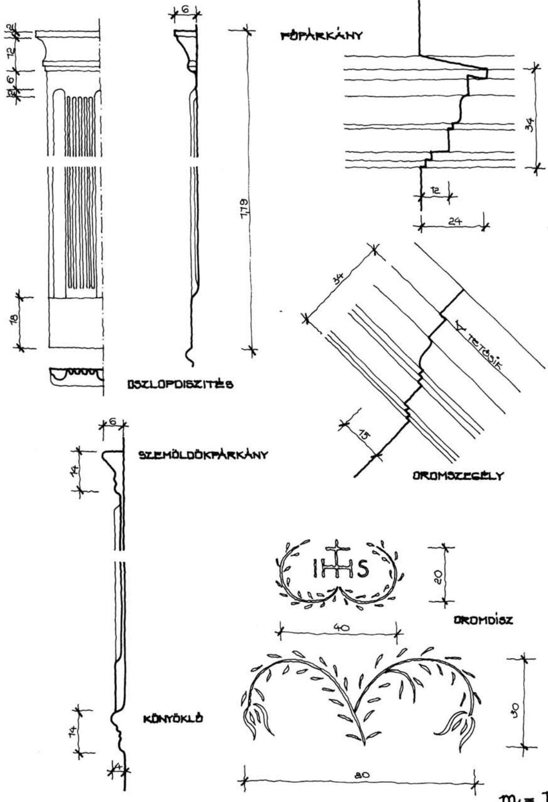
V/b. A Nagyráczt utca 20. alatti lakóház részletrajzai.
