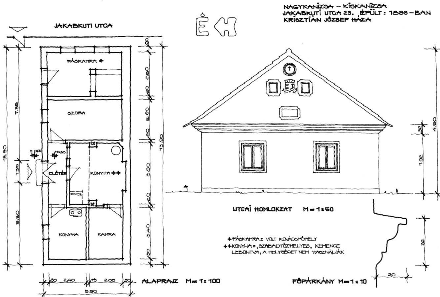
IV. A Jakabkúti utca 23. alatti ház homlokzata és alaprajza.
