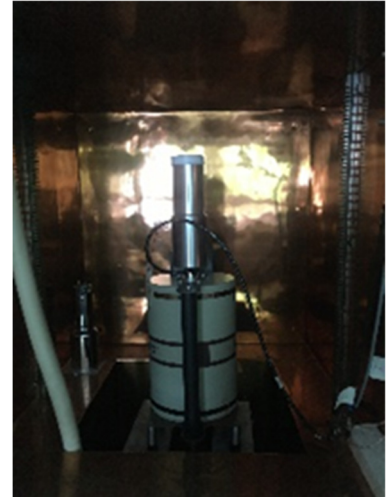
ORTEC Model GEM C40 detector
