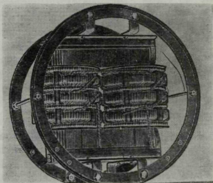
Egyfázisú oszlopos vasmagvú transzformátor (1890)
