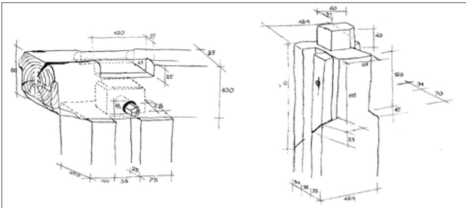
4. kép. Egy talpas-vázás, rólásos sertésól folyógerendájának és sarokoszlopjának kapcsolódása. Jól látszik a csap az oszlop tetején, és a nut, vagyis függőleges vajat az oldalán (A szerző rajza)
