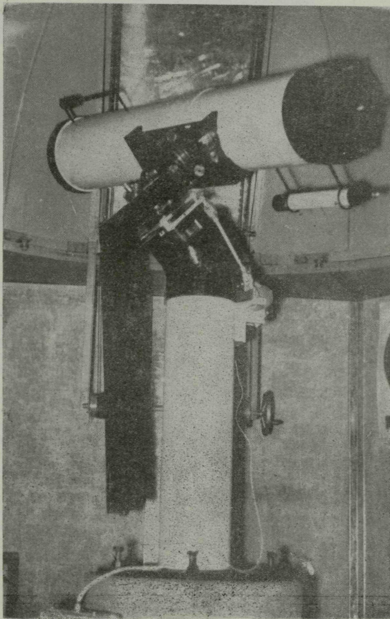
A három méter magas távcső a padozatból kiemelkedő acéllapos betontömbön.
