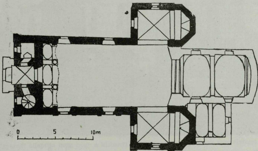
A jánosbócsai templom alaprajza. A feketével jelölt részek román koriak.
