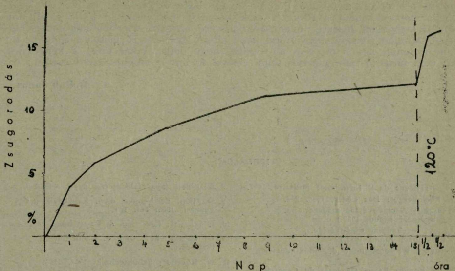
A mikropórusos gumitalp zsugorodása 15 napi pihenés és 1 órás hőkezelés alatt.
