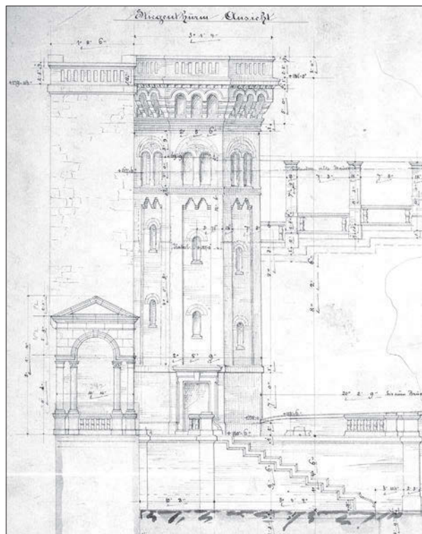
6. kép. A Lépcsőtorny keleti homlokzata a 2. rész 4. számú tervlapról, Forster Központ Tervtára
