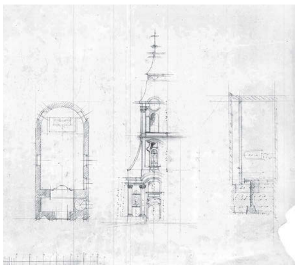
21. kép. A kastélyparkban álló kápolna alaprajza, nyugati homlokzata és hosszmetsete. Ybl Miklós ceruzás vázlatrajza, 1854–1860. BFL-XV.17.f.331.b-40/10.
