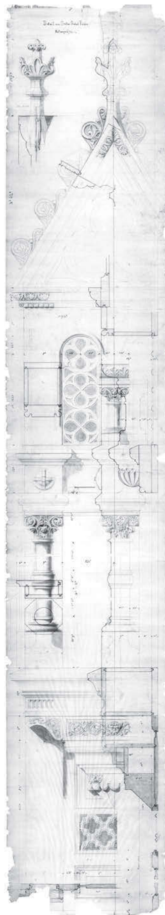
9. kép. Orgonaház oldaloromzati részletrajza. BFL XV.17.f.331.b-47/92.
