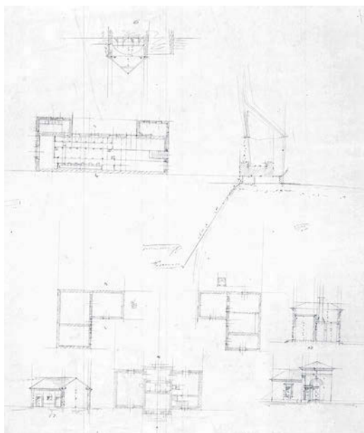
31. kép. Az egykor a kastélyparkban álló, lebontott növényház, valamint a három épületből álló kertészlak helyszínrajzai, alaprajzai, homlokzatai és metszetei. Ybl Miklós ceruzás vázlatrajza, 1854–1860. BFL-XV.17.f.331.b-40/7.
