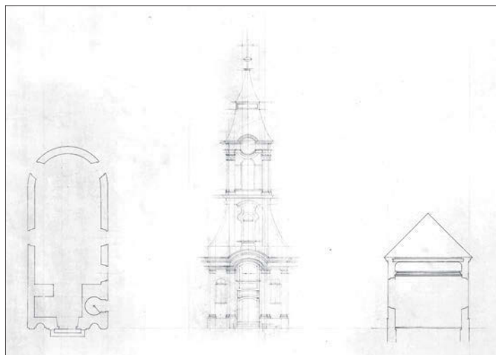
22. kép. A kastélyparkban álló kápolna alaprajza, nyugati homlokzata és keresztmetsete. Ybl Miklós vázlatlatterve, 1854–1860. BFL-XV.17.f.331.b-40/11.
