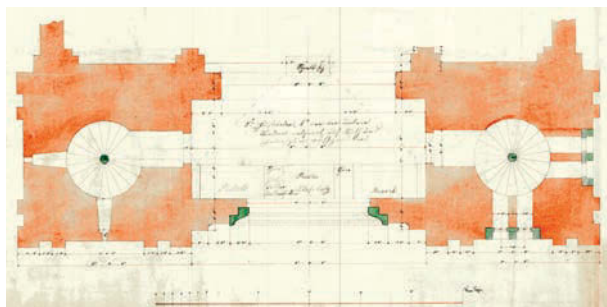
5. kép. Kaztatalaprajz. Játszóasztal a mellvédbbe tervezve. BFL 4/26.
