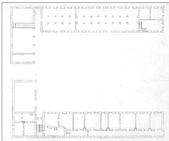
12. kép. A hátsó udvart körülvevő épületek alaprajza. Ybl Miklós vázlatterve, 1854–1860. BFL-XV.17.f.331.b-40/6.
