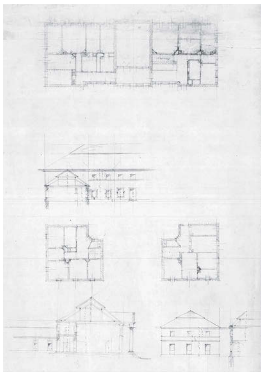
2. kép. A főépület és a pavilonok emeleti alaprajza, első udvari homlokzatokkal és metszetekkel. Ybl Miklós ceruzás vázlatrajza, 1854–1860. BFL-XV.17.f.331.b-40/2.
