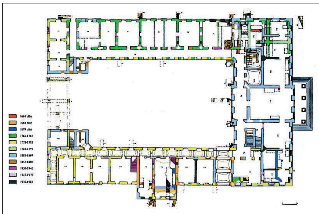
6. kép. A kastély földszinti periodizációs alaprajza.
