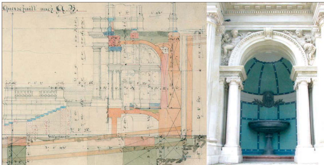
10. kép. A Gloriette medence téri metszete a 13. számú tervlapról, BTM Kiscelli Múzeum, Építészeti Gyűjtemény. Archív fotográfia, FSZEK Budapest Gyűjtemény
