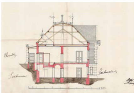
13. kép. Fest Vilmos villájának metszete. BFL XV.17.a 302 BMT 615/d.
