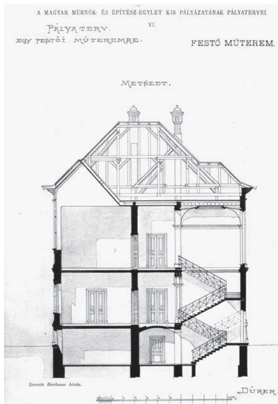
4. kép. Bierbauer István nyertes terve a Festőműterem-pályázatra, Építő Ipar , 12. 1888. Mellékletek
