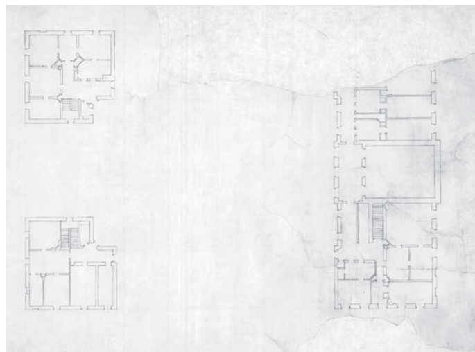
3. kép. A főépület és a pavilonok emeleti alaprajza. Ybl Miklós vázlatterve 1854–1860. BFL-XV.17.f.331.b-40/3.
