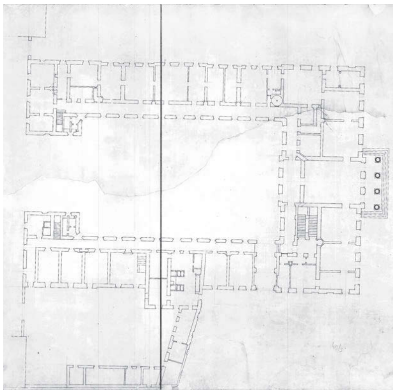
25. kép. A kastély földszinti alaprajza a konyhához csatlakozó, egykori cselédszárny ábrázolásával. Ybl Miklós vázlatterve, 1854–1860. BFL-XV.17.f.331.b-40/3.
