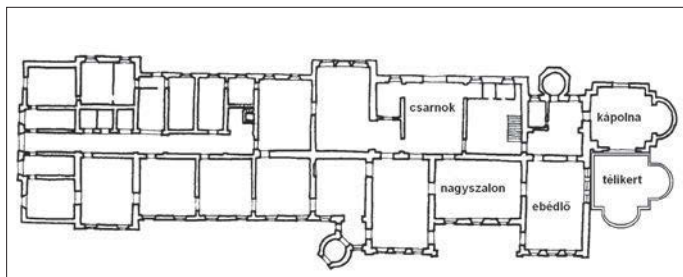
10. kép. Zsombolya, Csekonics-kastély. Ybl Miklós, 1869–1870. Földszinti alaprajz. BFL XV. 331. 31/5.
