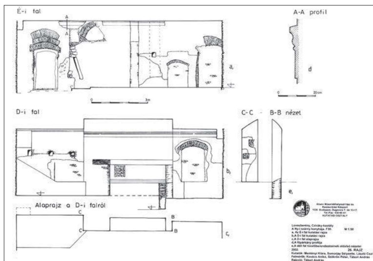
24. kép. A nyugati szárny konyhájának kutatási rajzai. Kutatási dokumentáció, 1997–2002
