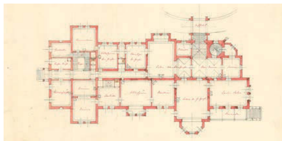
11. kép. Szabadkígyós, Wenckheim-kastély. Ybl Miklós, 1875–1879. Földszinti alaprajz
