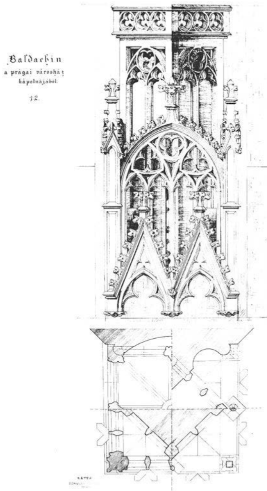
2. kép. Kremer Frigyes másodéves építészhallgató rajza a Publikationen der Vereines Wiener Bauhütte , 3. 1864. II. köt. 80. tábla alapján, 1908. Budapesti Műszaki és Gazdaságtudományi Egyetem, Építészettörténeti és Műemléki Tanszék Rajztára
