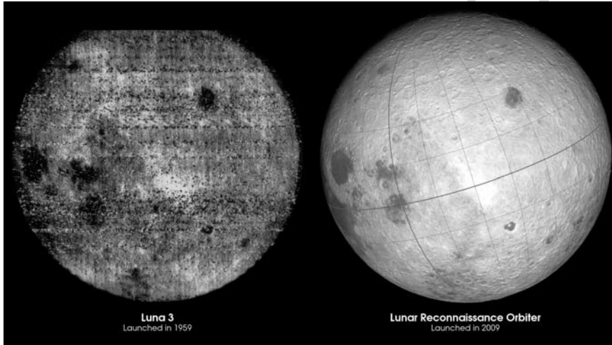
A Hold túlsó oldala a Luna-3 és az LRO felvételei alapján
