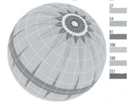
A TESS űrtávcső a teljes égbolton az egyes régiókat különböző időszakokon keresztül képes vizsgálni. A legrövidebb időszakok az ábrán látható gömb „közepes szélességein” állnak rendelkezésre, a megfigyelési időszakok a pólusok felé közeledve az átfedések miatt nőnek (NASA CC BY)
