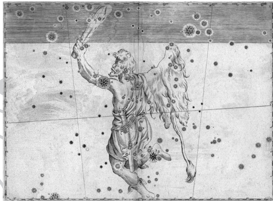
Az Orion csillagkép Bayer Uranometriájában. A fényesebb csillagokat a görög ábécé betűivel jelölte, a Betelgeuze lett az Orion alfája, az \alpha Orionis
