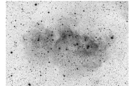
Szántó Szabolcs felvétele a Lélek-ködről (114/450 T, Canon EOS450D, 77x600 s ISO 1600)
