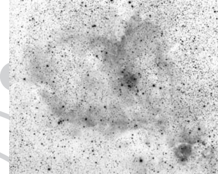
Lubai Csaba fotója a Szív-ködről (8 L, CentralDS Astro40D, 48x240 s, ISO 1000)
