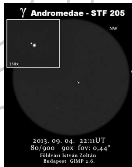
A γ And, STF205 Földvári István Zoltán észlelése szerint. 8 L, 90x
