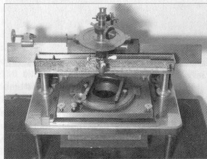
Gothard Jenő fotólemez kimérésére használt komparátora (1888) az ELTE Gothard Observatórium állandó kiállításán
