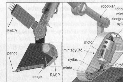
A robotkar végén lévő berendezés (balra), és azon a fűrófej kinyagított környezete (jobbra)
