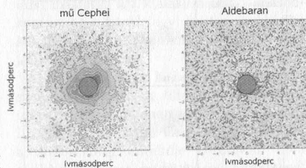
A \mu Cep és az Aldebaran körüli infravörös sugárzás eloszlása. Az Aldebaran esetében a pontszerű csillag körül nem mutatható ki semmilyen többlet. A középben látszó szürke kör a műszer diffrakcióhatártól felbontását illusztrálja
