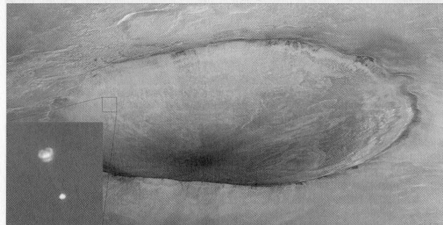
Az ereszkedő Phoenix az MRO felvételén, háttérben a 10 km-es Heimdall-kráterrel, amelytől 20 km-re landolt. A fotó készítésekor az MRO 760 km-re volt a Phoenixtől
