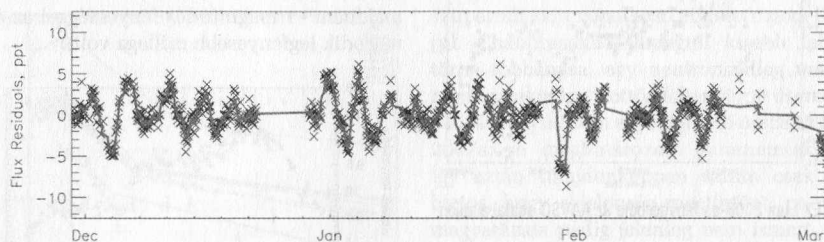
Három hónapnyi fénygörbe a \beta UMi SMEI-adataiból. A függőleges tengelyen a fluxus változásai vannak ezredrésznyi egységekben feltüntetve
