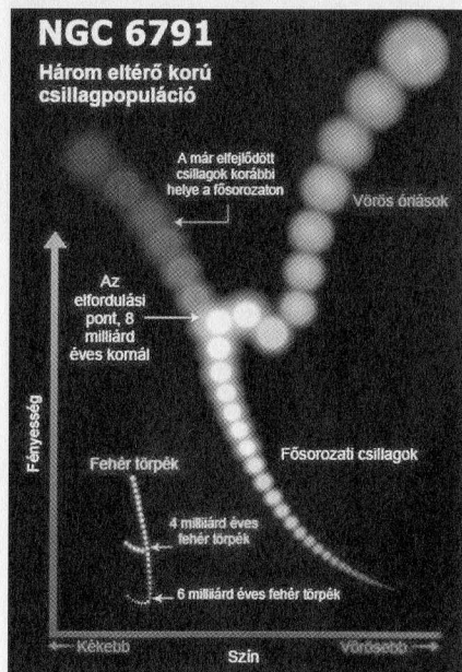
Az NGC 6791 szín–fényesség–diagramja, rajta a szövegben említett, a csillagfejlődés különböző állapotaiban lévő objektumokkal (STScI)
