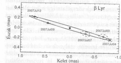
A \beta Lyrae relatív pályájának legjobb illesztése. Középen fekete körrel jelölve található a főkomponens, míg a pálya képzeletbeli vonalán a különböző időpontokban látható mellékkomponenszt üres kör szimbolizálja a hozzá tartozó hibahatárokkal (szaggatott vonalú kör). A pálya felső része van hozzánk közelebb, az inklináció közel 90 fok. [M. Zhao és munkatársai]
