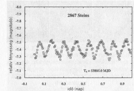
A 2867 Steins kisbolygó fényváltozását több cikluson keresztül mérte ki a Rosetta OSIRIS NAC műszere 2006. március 11-én (kép: Rosetta OSIRIS kutatócsoport)
