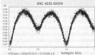
Egy \beta Lyrae típusú „névtelen” fedési kettős jellegzetes fénygörbéje az egyenlőtlen mélységű minimumokkal és a szinte folytonos fényváltozással. [K. V. Sokolovsky, Sternberg Astronomical Institute, Moszkva]
