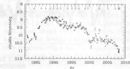
Az R127 vizuális, V és szűrős fénygörbéje 1982 és 2008 között
