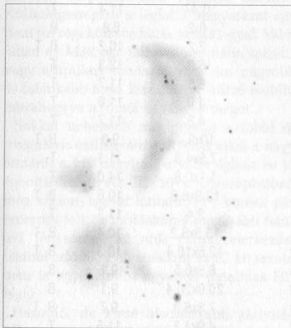
Az Antares körüli ködkomplexum Kiss Péter kis Dobson-távcsövével. 10 T, 16x, LM 4,5 fok. Észak fent, kelet balra van
