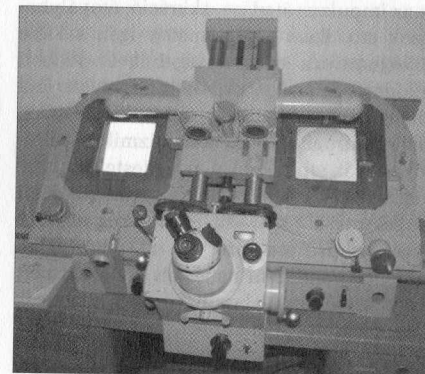
Az MTA KTM CSKI Zeiss sztereokomparátora, amellyel egybeként a Schmidt-lemezeket mérik ki
