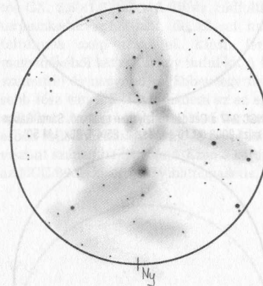
Kavargó gázfilamentek az IC 1470 körül, a Sharpless 156-ban. Sánta Gábor rajza 2008.08.31-én készült 220/1200-as Dobson-távcsővel, 133x nagyítással. A LM mérete 25'
