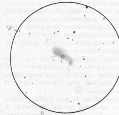
Az ajánlati NGC 6907-ben robbant SN 2008fq, valamint a galaxis spirálkarja mögött látszó háttérgalaxis (NGC 6908) nagyszerű látványt nyújtott Tóth Zoltán számára. 50,8 T, 273x, 16". A rajz 2008.09.28-án készült
