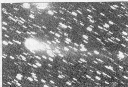
A Broughton-üstökös hosszú porcsóvája Csák Balázs és Sánta Gábor augusztus 6-ai, 20 perces felvételén. (40 T + CCD, LM= 6'x9')
