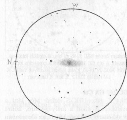
Tóth Zoltán rajza a különleges Cygnus-beli galaxisról, az NGC 7013-ról 2008.09.05-én készült, 50,8 T-vel, 409x-es nagyítással. A LM mérete 11'
