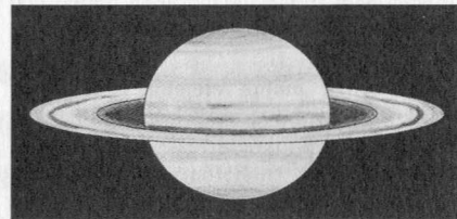
Ambrus Ádám ilyennek látta látta a Szaturnuszt 2008. május 14-én. Rajza 25,4 cm-es Newton segítségével készült
