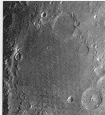
A Mare Nectaris Ladányi Tamás felvételén
