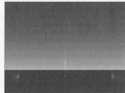
Szimulátor szoftverrel készült kép naposzlopról
