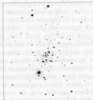
Az NGC 7419 NY Cep Kovács Attila digitális felvételének részletén. ISO 800, 6x3 perc expozíció, 2008.10.05. A LM 16'x14'. A keleti irány kissé jobbra felfelé esik
