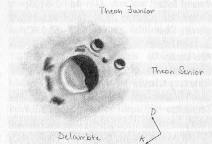
A Delambre-kráter. Klimaj Renáta a Polaris Csillagvizsgáló 20 cm-es Dobsonjával készítette ezt a rajzot
