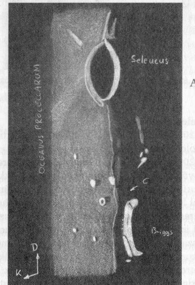
A Seleucus-kráter és a sötétségből éppen kibukkanó Briggs-kráter Görgei Zoltán rajzán...
