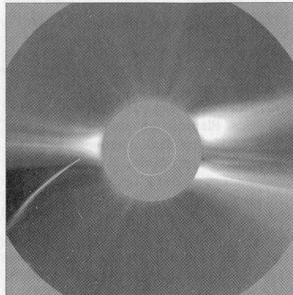
A SOHO napkutató szonda híres „karácsonyi üstököse”. A SOHO-6 üstökőst ábrázoló felvétele LASCO C2 koronagráffal készült 1996. december 23-án, 04:44 UT-kor
