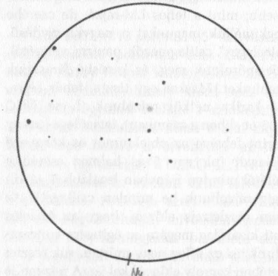
Az Andromeda-köd (M31) G76 jelű gömbhalmaza. 22 T, 300x (Sánta Gábor rajza)
