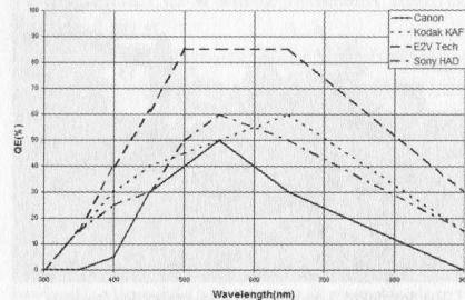
A Canon CMOS szenzorának és néhány elterjedtebb, csillagászati kamerákban használt CCD chip kvantumhatásfokának összehasonlítása
