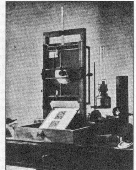
Weinek nagyítóval felszerelt tartóállványa, melynek segítségével rajzait készítette
