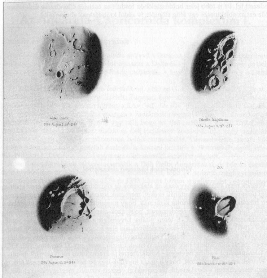
Néhány briliáns Weinek-rajz a prágai csillagvizsgáló publikációiból
