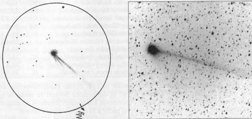
Március 8-án hajnalban Horváth Tibor és Tuboly Vince, valamint Sánta Gábor egy órán belül észlelte a Pojmanski-üstökösöt
