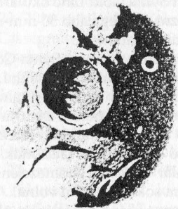
Az Archimedes-kráter vázlatrajza (jobbra) és teljesen kidolgozott rajza
