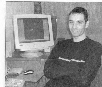
Cikkünk szerzője „észlelőhelyén”, a számítógépénél. A monitoron egy SOHO-felvétel látható
