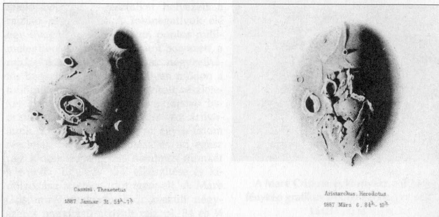
Weinek-rajzok közismert alakzatokról
