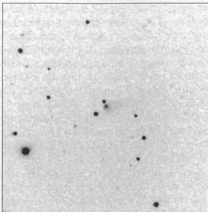
A C/2003 WT42 március 20-án este Horváth Tibor és Tuboly Vince 6 perces CCD-felvételén. A kép 8,6x8,6 ívperces égeterületet ábrázol
