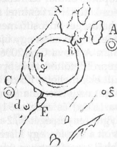
Az Archimedes-kráter vázlatrajza (jobbra) és teljesen kidolgozott rajza
