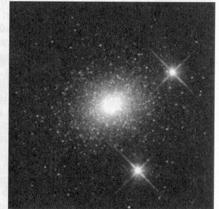
Az Andromeda-galaxis legfényesebb, G1 jelű gömbhalmaza a HST felvételén
