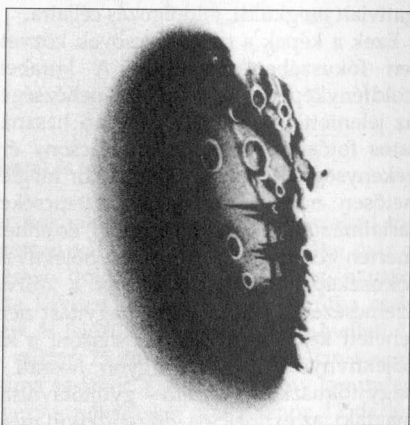
Távcső mellett készült rajz, ugyancsak a Mare Crisiumról (1884. március 14., 15:30–16:30)
