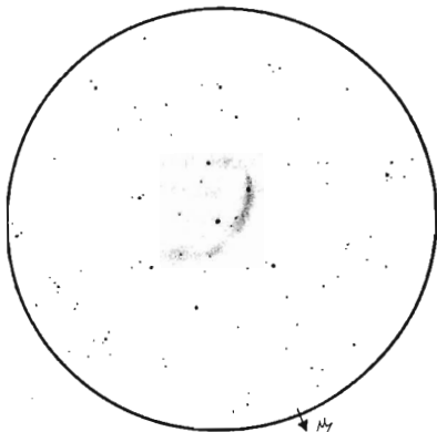
NGC 6888
