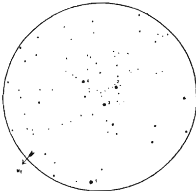
NGC 6910
