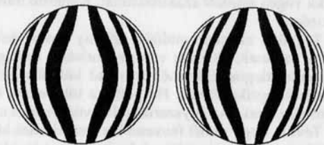
A Ronchi-rácsteszt. Balra: alulkorrigált felület, jobbra: tökéletes felület rácsképe
