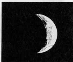
Balra: 2002.12.12. 05:15 UT, 20C, 180x, neutrál III szűrő, (Polaris Csillagvizsgáló, Hollósy Tibor); jobbra: 2002.12.12. 05:30 UT, 20C, 180x, neutrál III szűrő, (Polaris Csillagvizsgáló, Bánhalmi Balázs)
