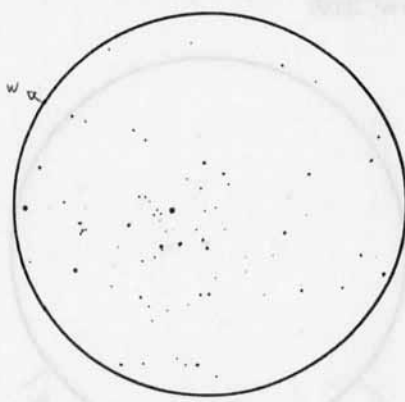
NGC 1027
