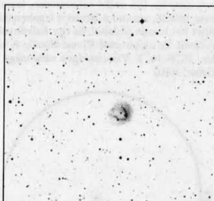
DSS-felvétel (PK 101.8+08.7)
