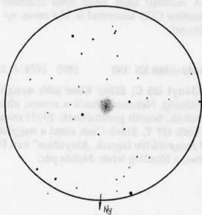
Czernik 13
