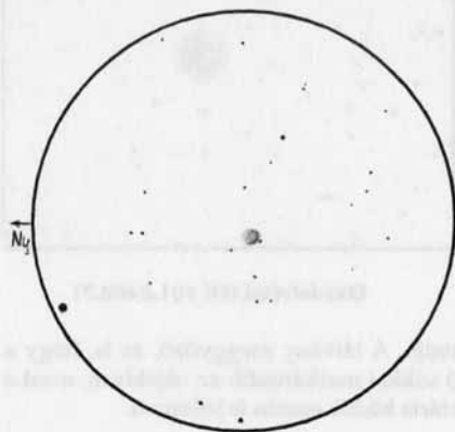
35,5 T, 263x, LM= 15' (Berkó Ernő)
