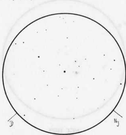
Fent: 35,5 T, CCD, 3,5'x4,5' (Berkó Ernő) Balra: 30,5 T, 169x, LM=17' (Kernya János Gábor)
