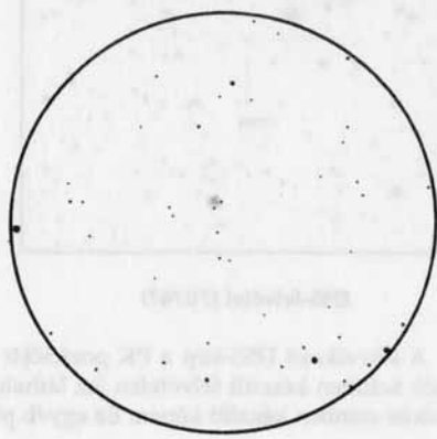
30,5 T, 169x, LM ~17' (Kernya János Gábor)
