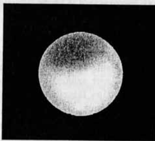
2002.05.02. 01:45 UT, 20 T, 167x, (Polaris Csillagvizsgáló, Hollósy Tibor)
