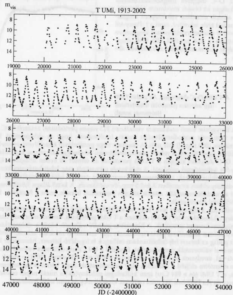
A T UMi teljes fénygörbéje (10-napos átlagpontok). A legelső panel szürke pontjai az AFOEV által gyűjtött V-szűrős CCD-méréseket mutatják
