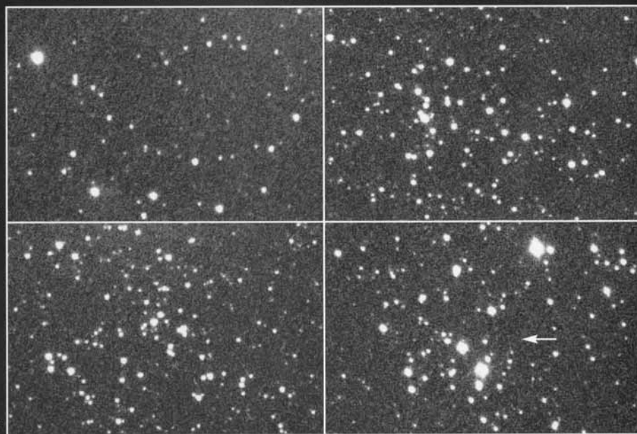
Galaxisok a Pegasus csillagképben: 1. NGC 7479, 2. NGC 7678, 3. NGC 7741, 4. NGC 7769 (balra), 7770 (jobbra fent) és 7771 (jobbra lent). Nyílthalmazok a Cepheusban és a Cassiopeiában: 5. Berkeley 93, 6. King 4, 7. Czernik 13, 8. Berkeley 63 (Berkó Ernő felvételei, 35,5 cm-es Newton, Amakam CCD – információk a Mély-ég objektumok című rovatban)
