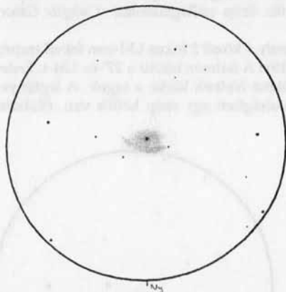
Van den Bergh 8
