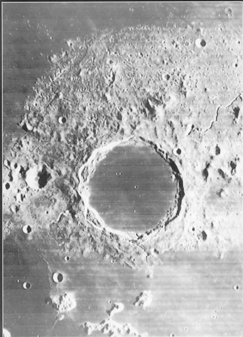
A Plato-kráter „felülnézetből”, a Lunar Orbiter 4 felvételén (bővebben lásd A Plato krátere i című cikkünket)
