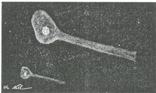
A kettészakadó Biela-üstökös J.H. Mádler könyvének illusztrációja szerint
