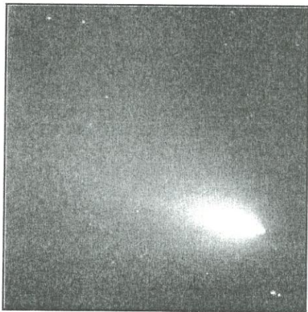
Balra: A felbomlása kezdetén lévő üstökös július 26-án. A képet M. Kidger készítette a La Palma-i 1 m-es Jacobus Kapteyn reflektorral. Jobbra: Augusztus 1-jén a 2,5 m-es Isaac Newton Telescope-pal már csak ennyi látszott az üstökösből. M. Kidger 4,5x4,5 ívperces területet megörökítő felvétele 100 másodperces expozícióval készült
