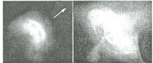
A Vela-pulzárt (balra) és a Rák-pulzárt (jobbra) övező szerkezet
