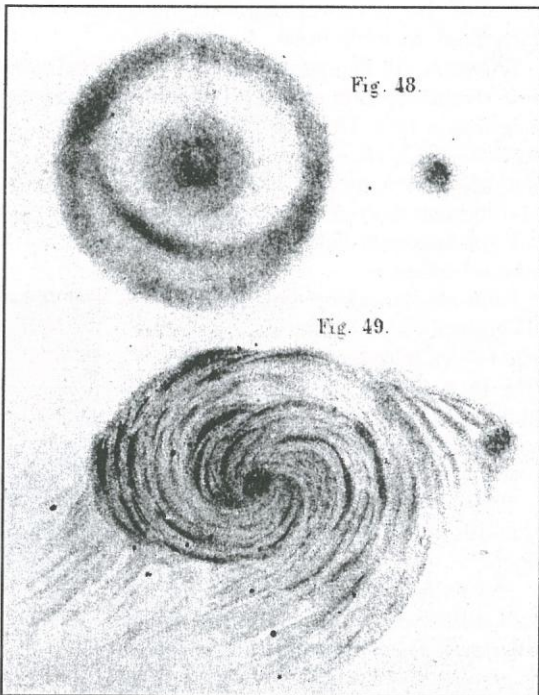
A Vadászebek spirális köde, ahogyan a 19. sz.-ban kis távcsővel (fent) és órástávcsővel (lent) látták
