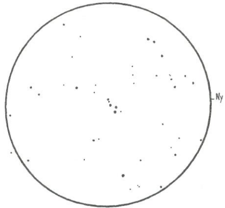
DoDz 6 (254/1525 refl., 47x, LM= 1°10')
