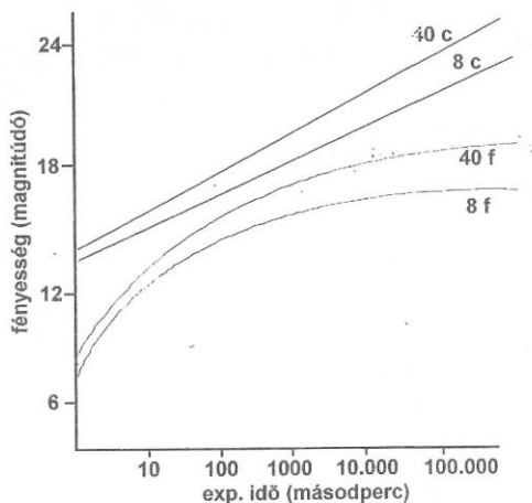
8 és 40 cm-es távcsövekkel elérhető határmagnitúdók különböző expozíciós idők mellett fotografikus és CCD technikával
