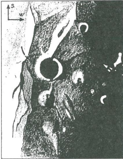
Arago \alpha és \beta dóm 1998.07.29. 18:35–19:10 UT Colong.= 341°03 200/1500 refl., 150x (Sánta Gábor)
