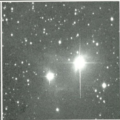
Fent balra a T Tauri reflexiós köde (NGC 1555) 1998.10.23. 03:15 UT
