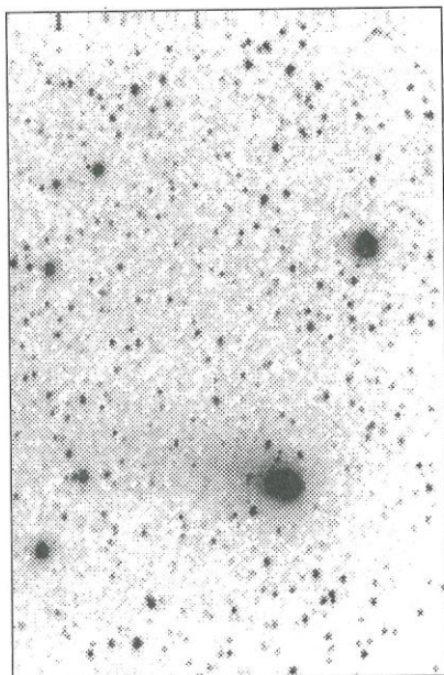
Balra: Sánta Gábor és Willand Péter CCD-képe a Giacobini–Zinner-üstökösről, 1998. okt. 10. 20:40 UT-kor, jobbra: ugyanezen észlelőpáros felvétele az 1998 K5 (LINEAR) üstökösről 1998. okt. 11. 01:45 UT-kor. A felvételek 28 cm-es Schmidt–Cassegrain-távcsővel és ST-6-os CCD kamerával készültek
