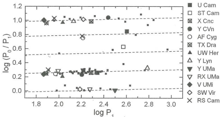
3. ábra. Periódusarányok a hányados nevezőjében levő rövidebb periódus függvényében
