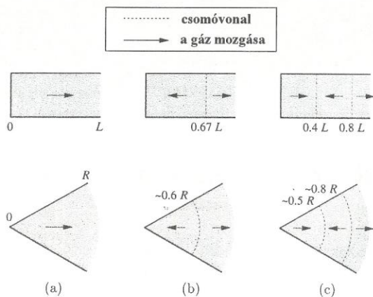
1. ábra. A sípban rezgő légoszlop és egy pulzáló csillag összehasonlítása. (a) alpmódus, (b) első felhang, (c) második felhang
