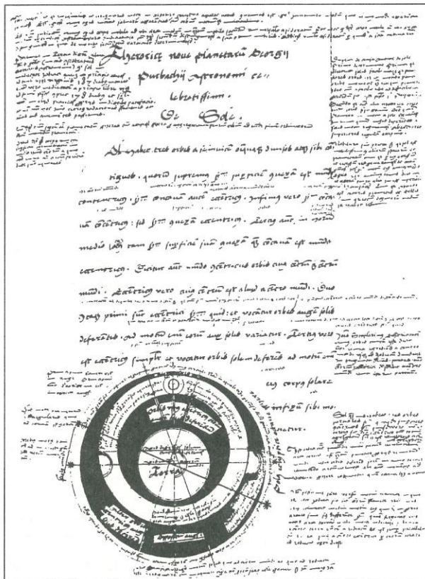
2. ábra. Peurbach elképzelése a bolygómozgásokról (mozgó modell képével)
