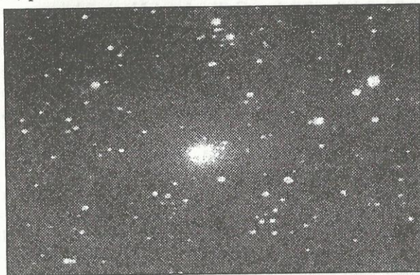
A Hyakutake-üstökös január 31-én, egy nappal a felfedezés után. A felvételt Takou Kojima készítette 25 cm-es Newton-reflektorral és ST-6-os CCD-kamerával. Az expozíciós idő 120 s.
