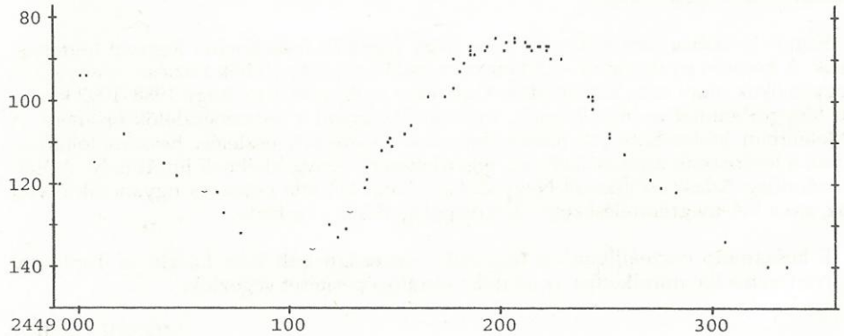
1611+38 W CrB
