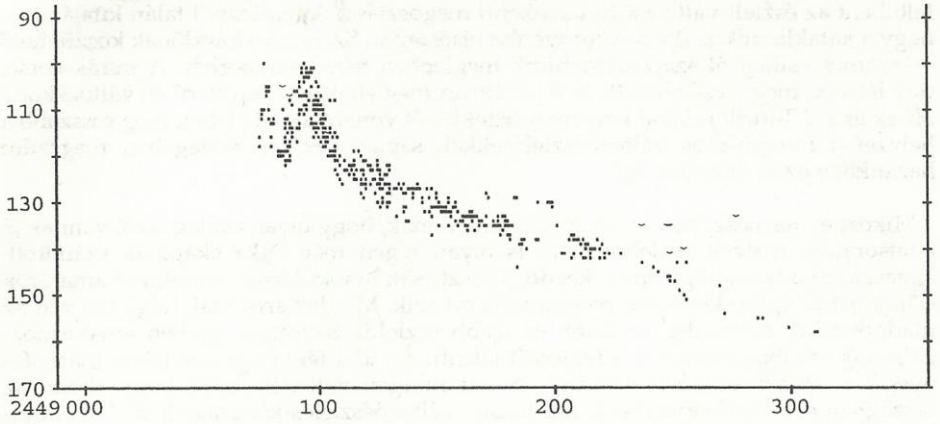
1908+01 V1419 Aql
