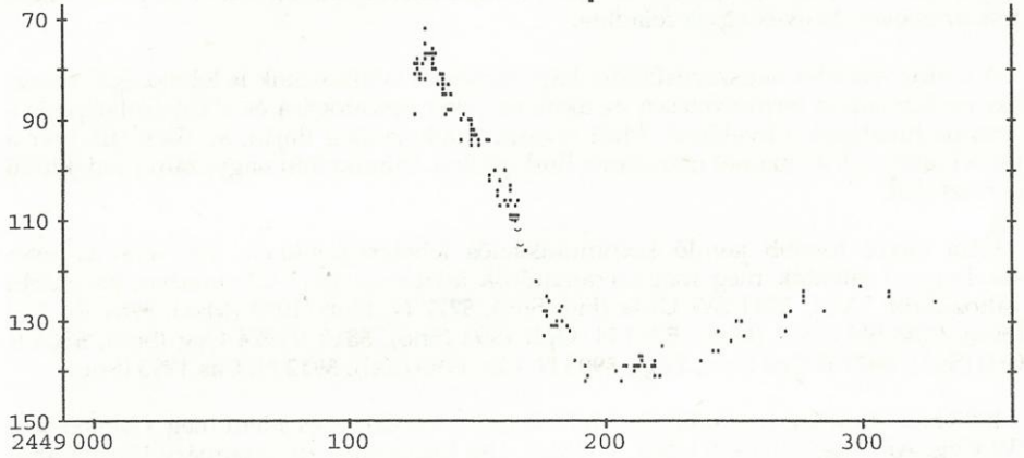
1908+01 V1419 Aql
