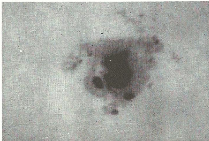
Szabadszemes napfoltcsoport 1993. március 10-én, 11:40 UT-kor. 110/1650-es Zeiss AS refraktor, 6,3-as pozitív nyújtás, Herschel-féle napprizma, ORWO MA 9-es film, 1/1000 s expozíciós idő (Farkas László).
