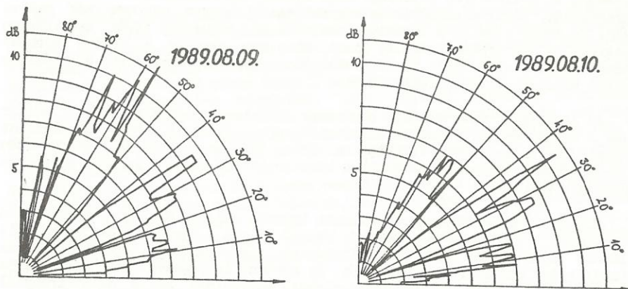
2. ábra: Az napzaj változása 94,7 MHz-en a Nap irányszögének függvényében déltől nyugatig (dél fent, nyugat jobbra)
