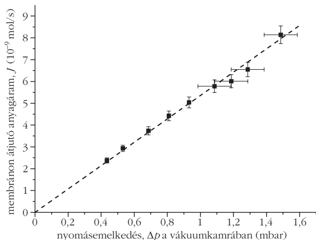
3. ábra. A membránon átfutó anyagáram és a vákuumkamrában mérhető nyomásemelkedés kapcsolata (125 \mu\text{m} vastag PTFE membrán, \text{H}_2 permeáció, szobahőmérséklet). A szaggatott vonal az origón átmenő, az adatpontokra illesztett egyenes, amelynek meredeksége megadja a (15)-ben szereplő k értékét.
