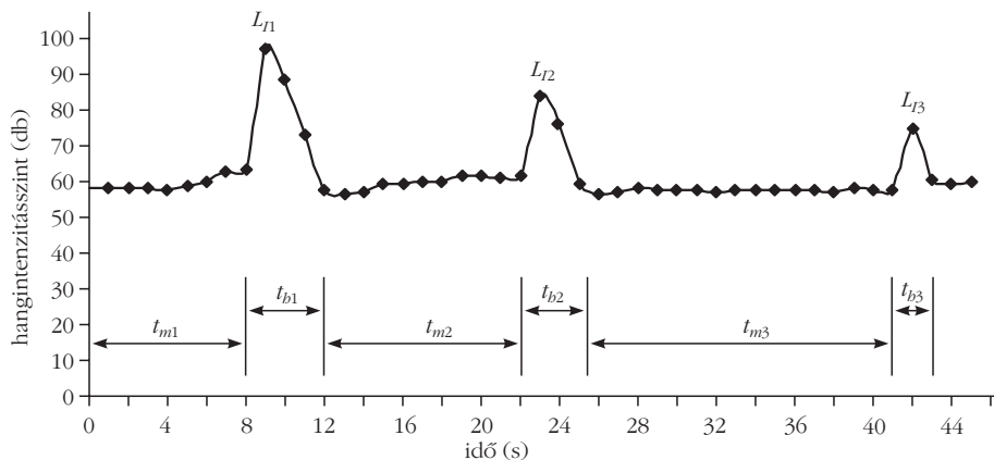
2. ábra. A kibocsátott hang intenzitása és hossza is csökken, ha nem hagyjuk visszahűlni a csövet. A rács a 400 mm-es üvegcső negyedrésznél helyezkedett el, az égőteltjesítmény körülbelül 270 W volt. (Ebben az esetben az egyik kísérlet után rögtön végrehajtottuk a következő mérést.)
