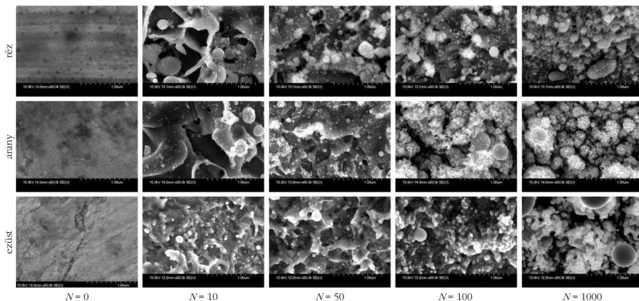
5. ábra. 190 mJ/cm² energiasűrűségnél különböző impulzusszám esetén kialakuló felületi struktúrák.
