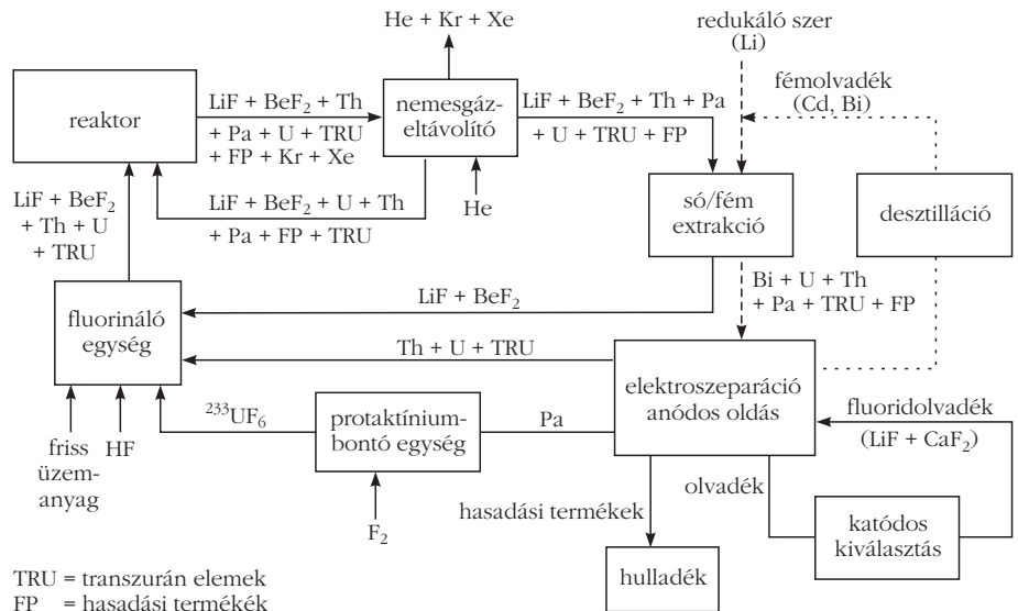
1. ábra. A sókezelés teljes folyamata.
