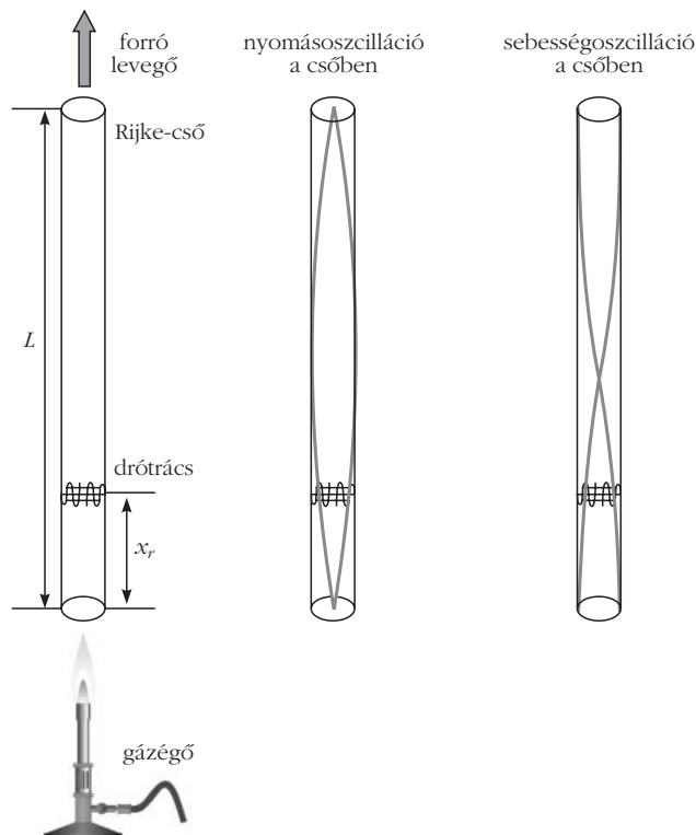
3. ábra. A Rijke-csőben az akusztikus nyomás és sebesség szemléltetése (alapharmonikus eset).
