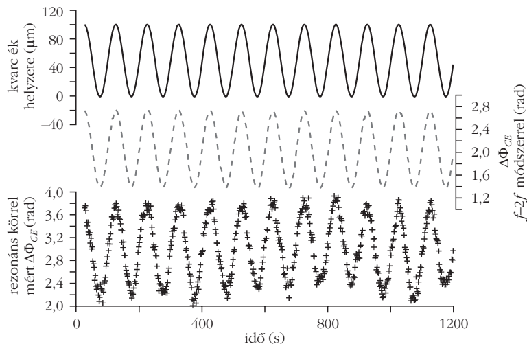
5. ábra. A rezonátoron belüli ékpár [3] egyik tagjának az optikai tengelyre merőlegesen, szinusz függvény mentén történt mozgásával kapott eredmények.
