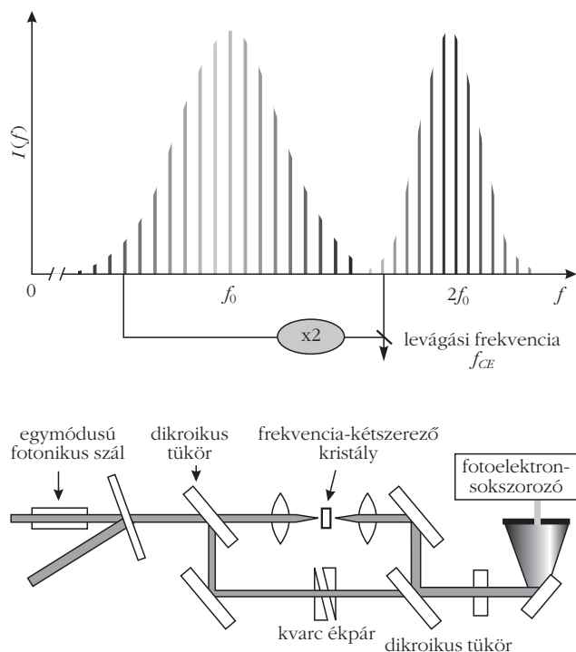
2. ábra. Az f - 2f interferencián alapuló mérés alapelve [2, 3].
