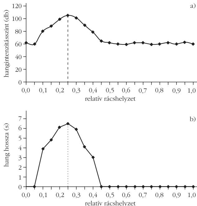
1. ábra. A relatív rácshelyzet x_r/L = 0,25 esetén lesz a hangintenzitásnak és a kibocsátott hang hosszának is maximuma. a) Hangintenzitásszint a relatív rácspozíció függvényében. b) Kibocsátott hang hossza a relatív rácspozíció függvényében. (A 470 mm-es részcsőben az égőteltjesítmény mintegy 350 W volt. A körülbelül 60 dB-es hangintenzitásszint az alapzajnak felelt meg.)
