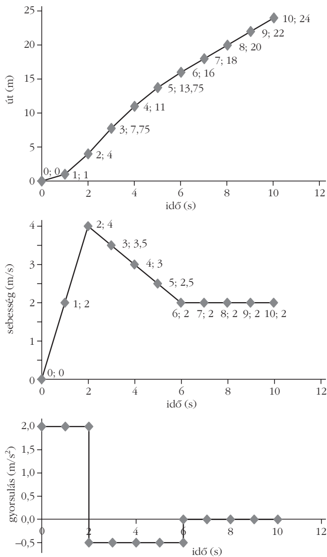
2. ábra. A mozgó testet különböző szempontból – gyorsulás-idő és út-idő (e kettőt vártuk el a tanulóktól), valamint középen az eredményeként megadott sebesség-idő – jellemző grafikonok.
