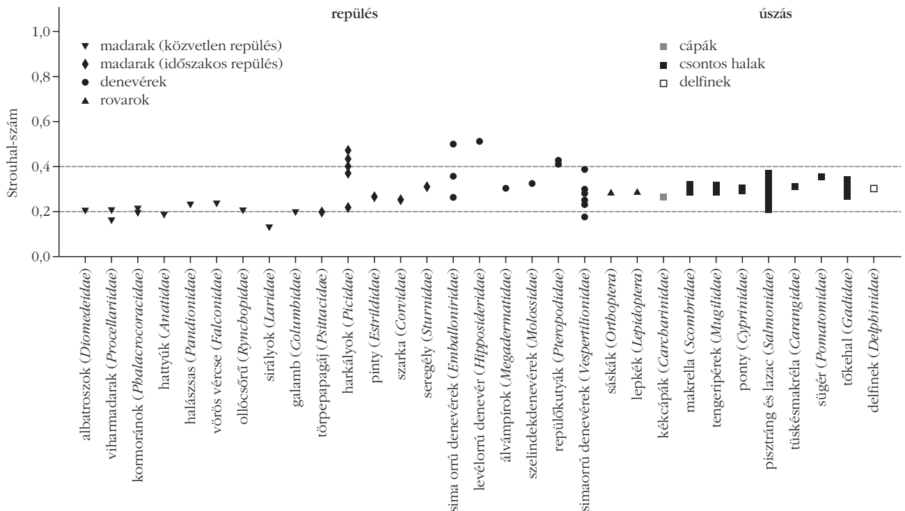
3. ábra. 42 madárfaj, denevér és rovar (valamint halak, delfinek) Strouhal-száma kitartó repülés (úszás) közben. Látható, hogy 0,2 < S < 0,4 [1]. A röpssebességhez közel (4-6 m/s) az álvámpír ( Megadermatidae ) Strouhal-száma 0,17 < S < 0,22 értéktartományba esik, amely kapcsolatban van a hatékonyabb szárnymozgással. A harkályfélék ( Picidae ) magas Strouhal-értéke ( 0,35 < S < 0,5 ) ugyancsak a szárnymozgásra vezethető vissza. A sirályfélék ( Laridae ) alacsony Strouhal-száma azzal magyarázható, hogy a levegőben alapvetően inkább siklómozgást végeznek.
