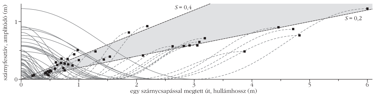
4. ábra. 42 madárfaj, denevér és rovar Strouhal-számának grafikus meghatározása kitartó repülés közben. A Strouhal-szám a szárnyfesztáv és az egy szárnycsapással megtett út hányadosaként adódik. Jól látható, hogy a repülő állatok Strouhal-száma általában a 0,2–0,4 meredekségű egyenesek közé esik [3].
