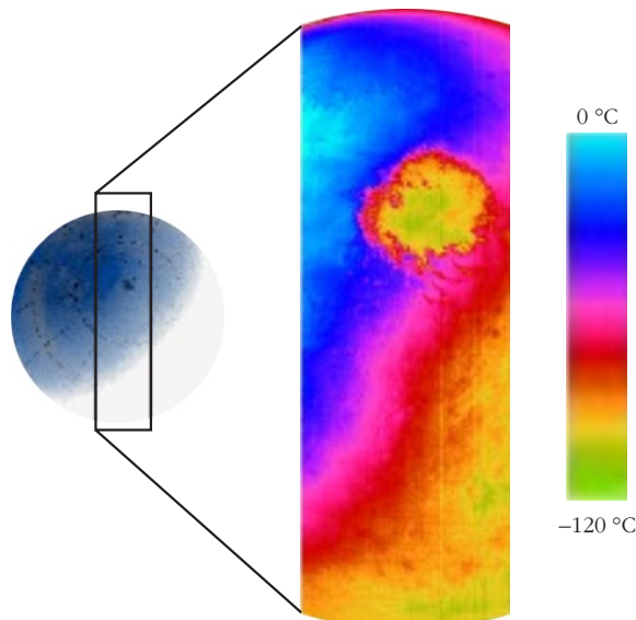
2. ábra. Égitest hőtérképe. (Forrás: http://www.fs121.com/channel/news/mars45.html )
