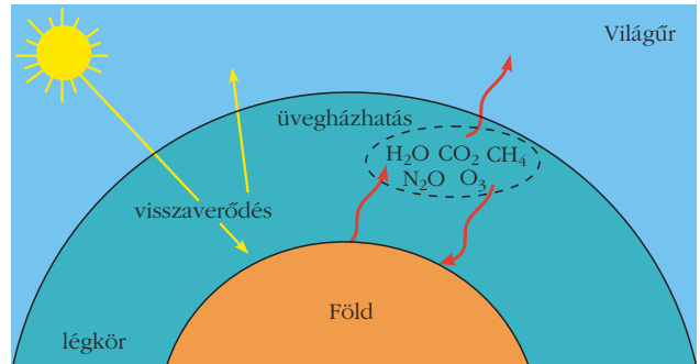
5. ábra. Egyszerű üvegházmodell. (Forrás: http://bildungsserver.hamburg.de/atmosphaere-und-treibhauseffekt/2069648/treibhauseffekt-natuerlich-artikel.html )
