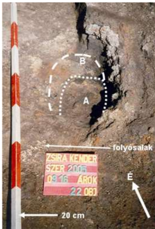
4. ábra. Az 1. kohó (Zsira, 22. objektum). A: a korábbi kohó medencéje; B: a későbbi, újjáépített kohó medencéje és oldalfala.
