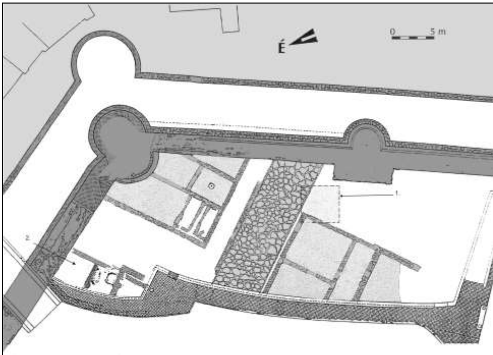
1. ábra. A Városház utcában feltárt épületek, 1. Tóth Sándor ásátásából származó ház helye, 2. Gömöri János által 2000-ben feltárt ház
