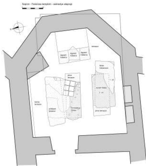
1. ábra. Sopron, ferences templom. A sekrestye ásatási alaprajza
