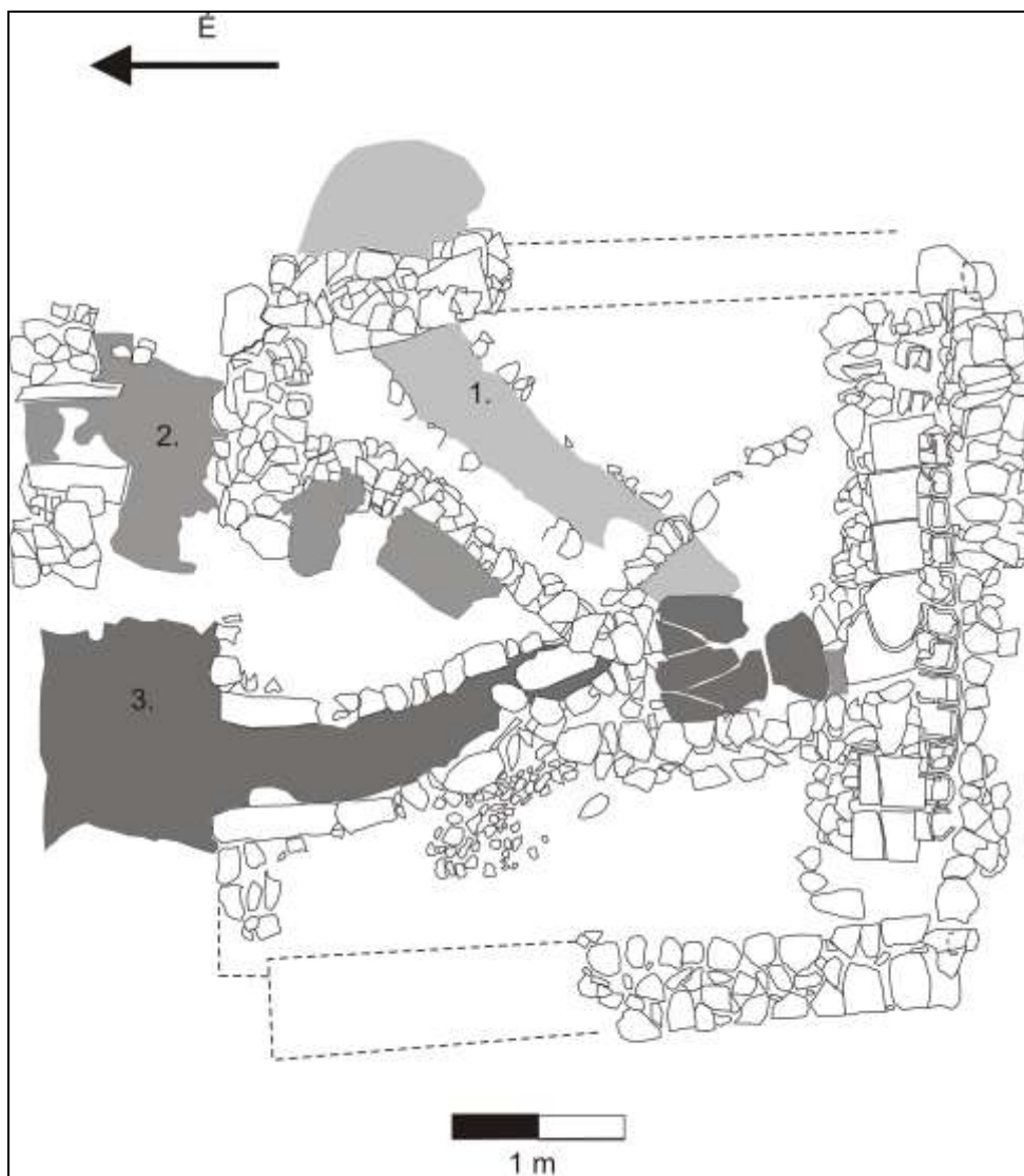
3. ábra. Az 5. századi ház alaprajza, a fűtőcsatornákkal; 1.: az első periódusú kemencéhez tartozó hamus felület és annak bekötése; 2.: második periódusú kemence faszenes része és a bekötő csatorna maradványai a kőlapokkal; 3.: harmadik periódusú kemencéhez tartozó hamus, paticsos felület, a bekötő csatorna és annak fedőlapja
