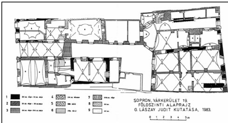
136–137 Sopron Várkerület 19. földszinti alaprajz G. László Judit kutatása, 1983.
