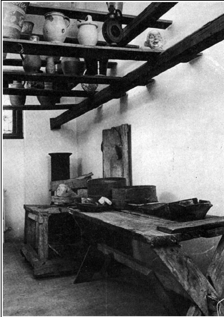
243 Fizekasműhely részlete, munkaasztal, XIX. századi korongpad, szárítók, XIX. század
