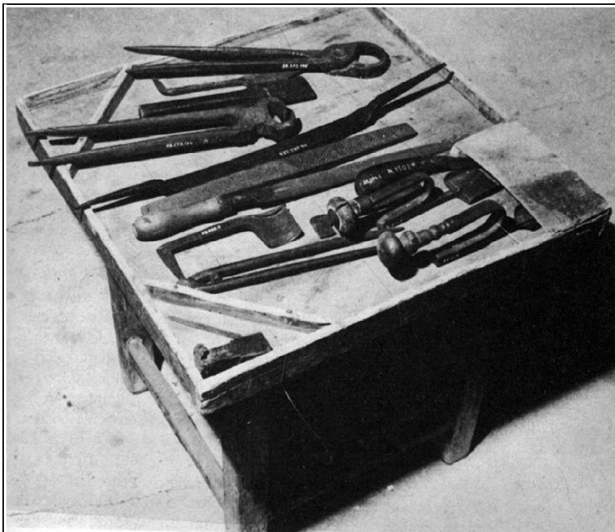
259A patkolóasztal szeszámái, XIX. század közepe
