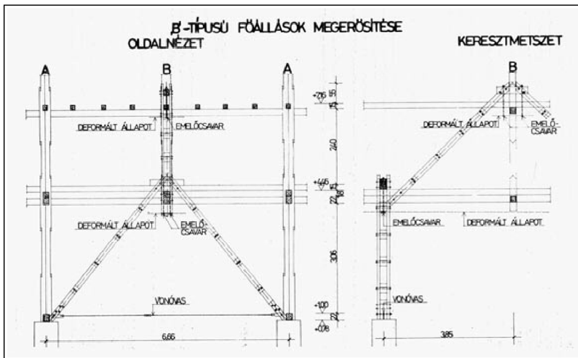
55. B"-típusú főállások megerősítése oldalnézet – keresztmetszet
