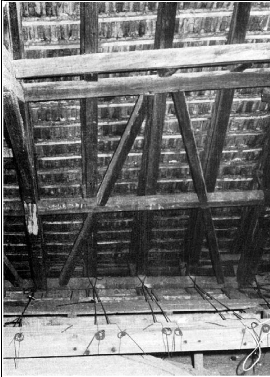
411. A veszélyes tetőszakasz visszakötése
