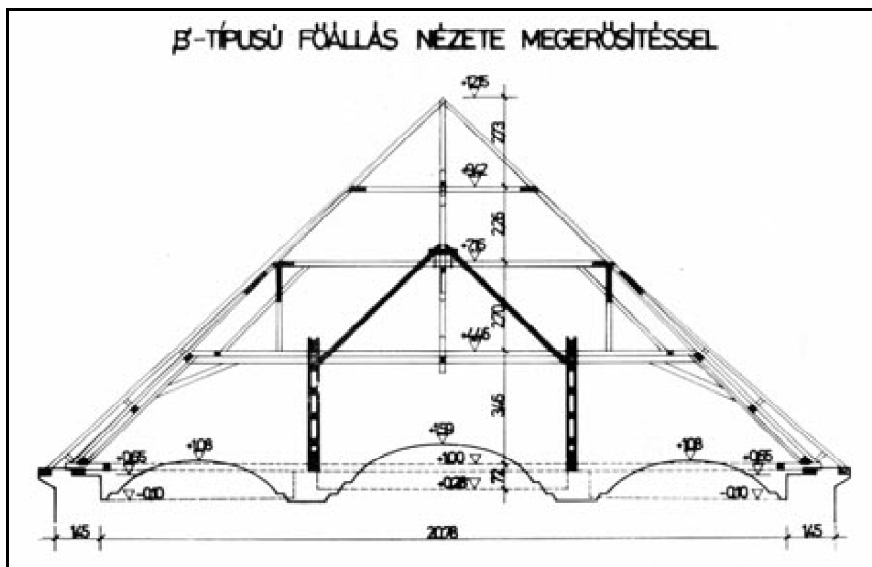
48. „B”-típusú főállás nézete megerősítéssel
