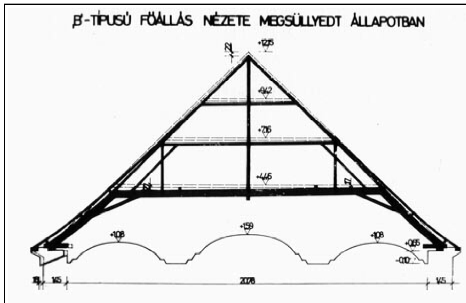
45.,B"-típusú főállás nézete megsüllyedt állapotban
