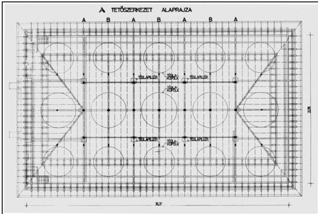
43A tetőszerkezet alaprajza
