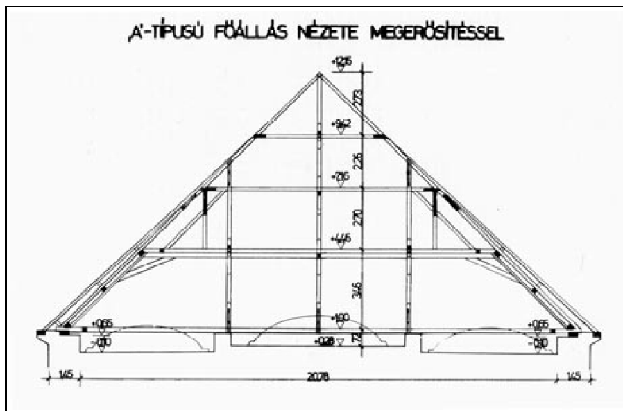
52. „A”-típusú főállás nézete megerősítéssel
