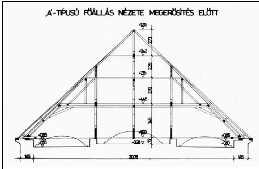
44.,A"-típusú főállás nézete megerősítés előtt
