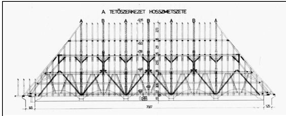
53A tetőszerkezet hosszmeteszete
