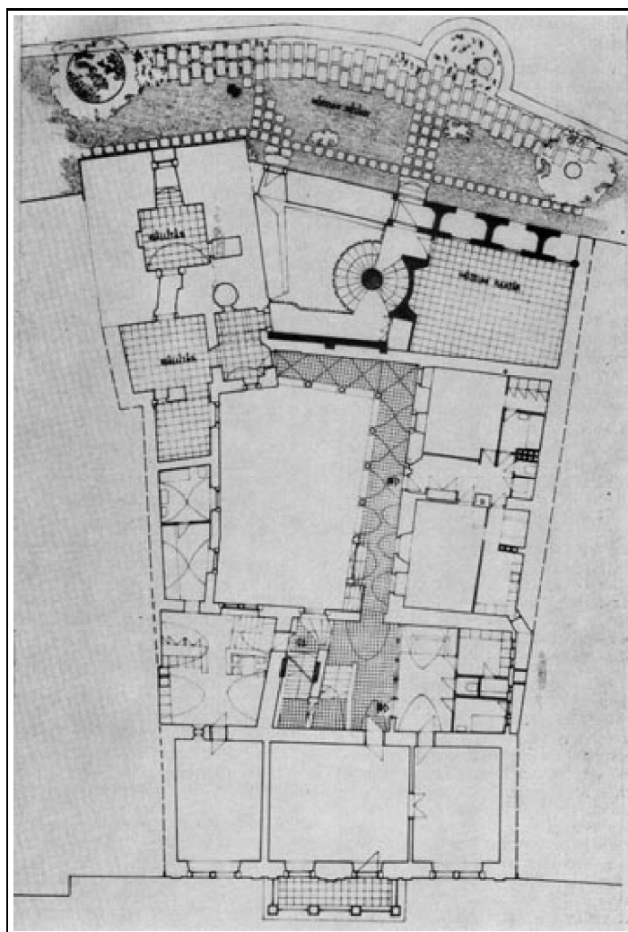
3252. Fő-tér 7. sz. emeleti alaprajza, felül az első városfal vonalában álló (lakó)-torony alsó szintjével
