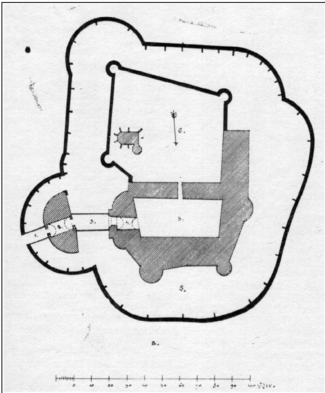
1531. A kaboldi vár helyszínrajza (Könyöki J. 1884. évi felvétele alapján): 1. Felvonóhíd; 2. Külső kapubástya; 3. Felvonóhíd; 4. Belső kapu; 5. Reneszánsz belső udvar; 6. Középkori várudvar; 7. Várkáporna; 8. Fallal körülvelt vizesárok
