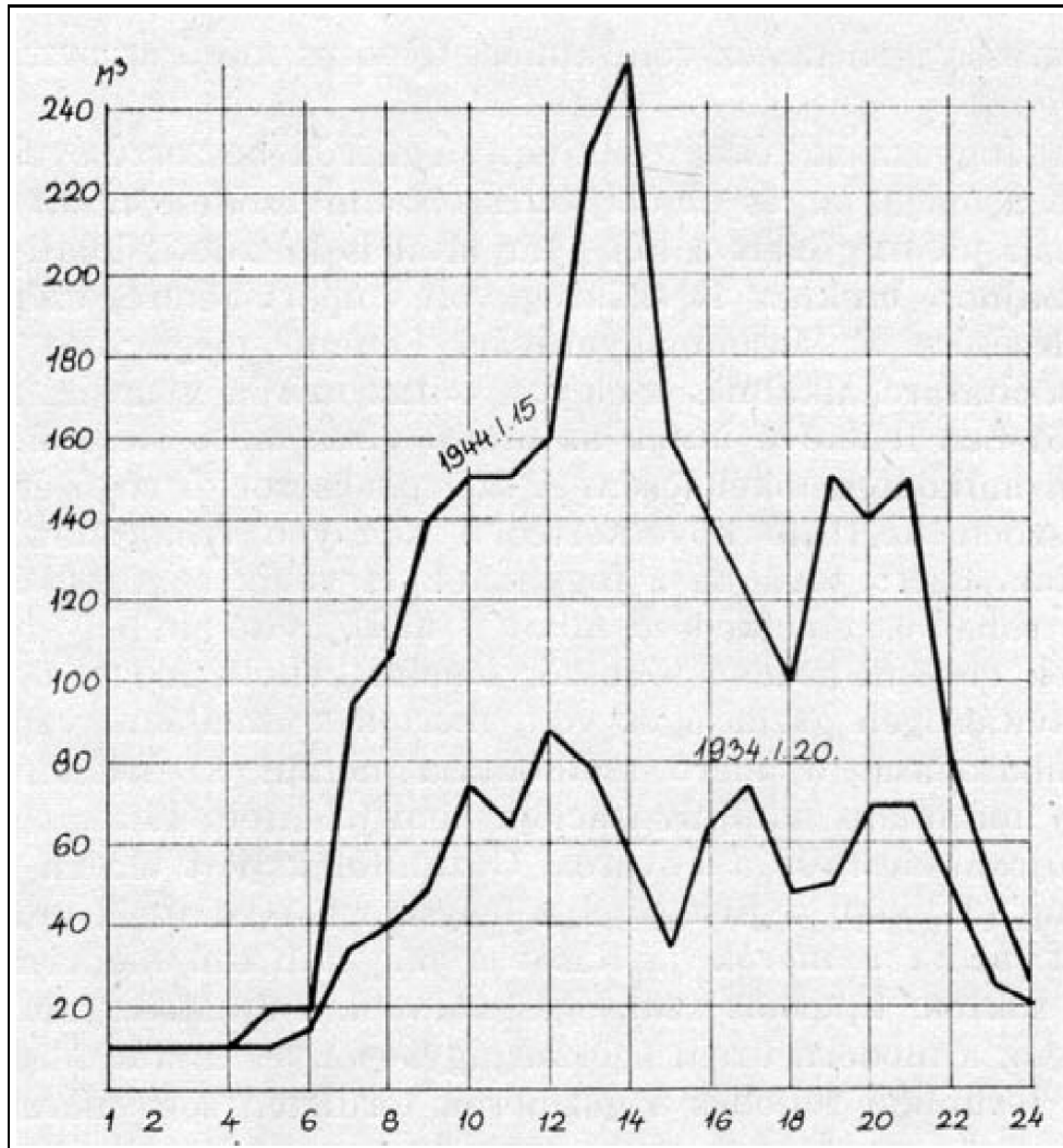
12732/a. Órákenti gázleadás (1934, 1944)
