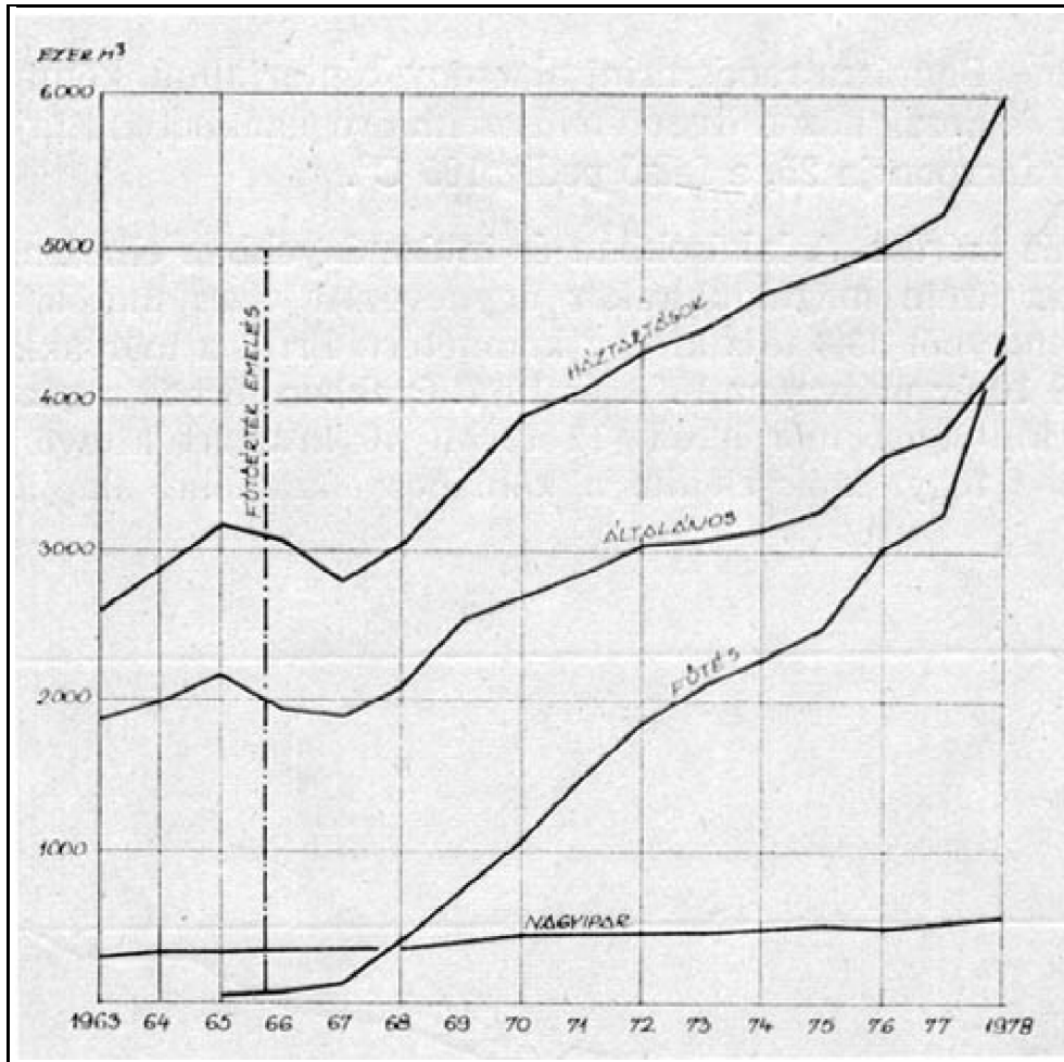
12631/a. A gázfogyasztás megoszlása (1963–1978)
