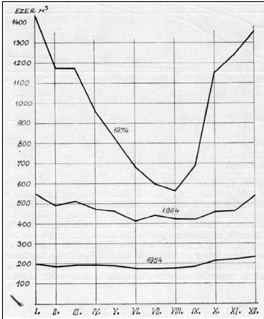
31/b. Havonkénti gázleadás (1954, 1964, 1974)
