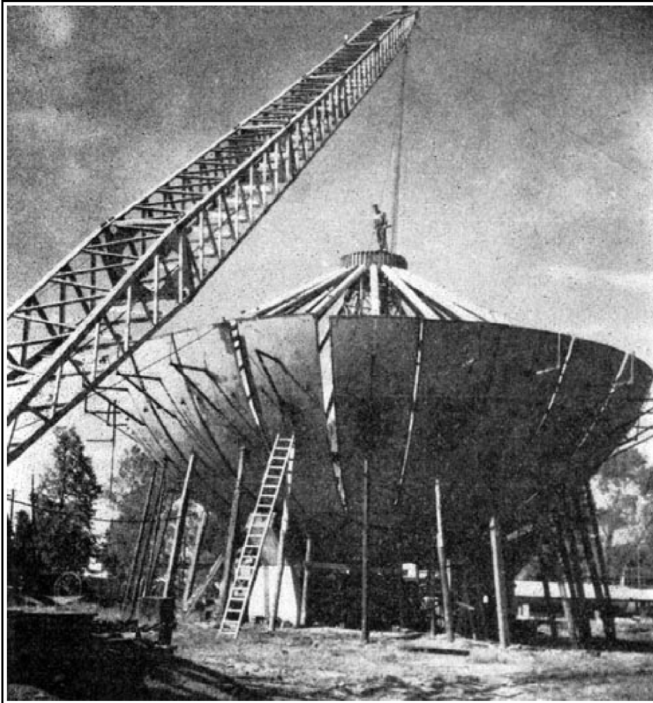
18. A gömbgáztartó szerelése (1965)
