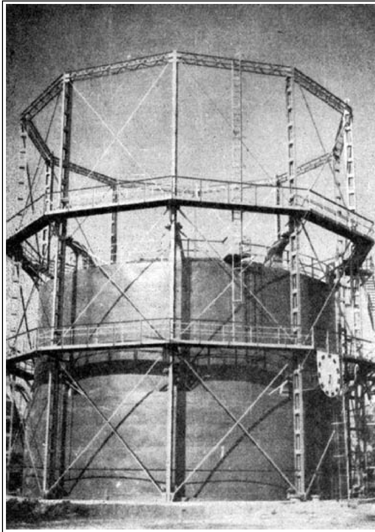
16. Az új, 4500 m 3 -es gáztartó (1955)
