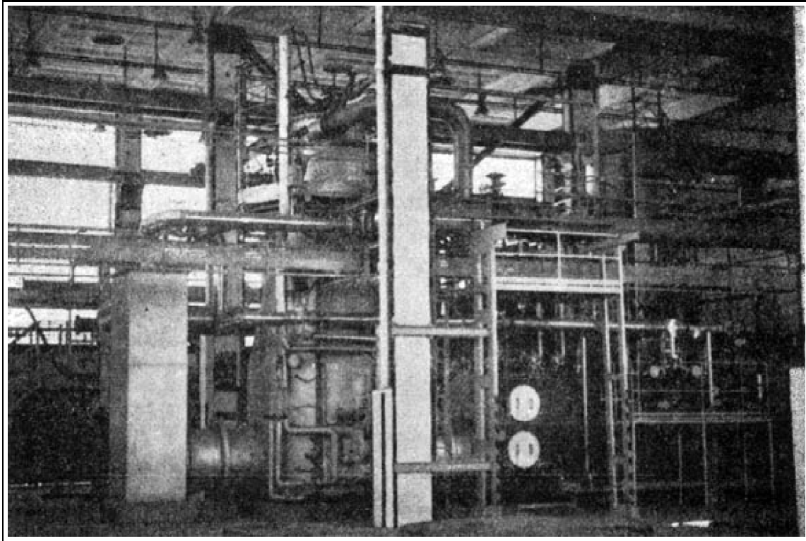
12328. Vízgőzös bontó az Ágfalvi úton (1975)
