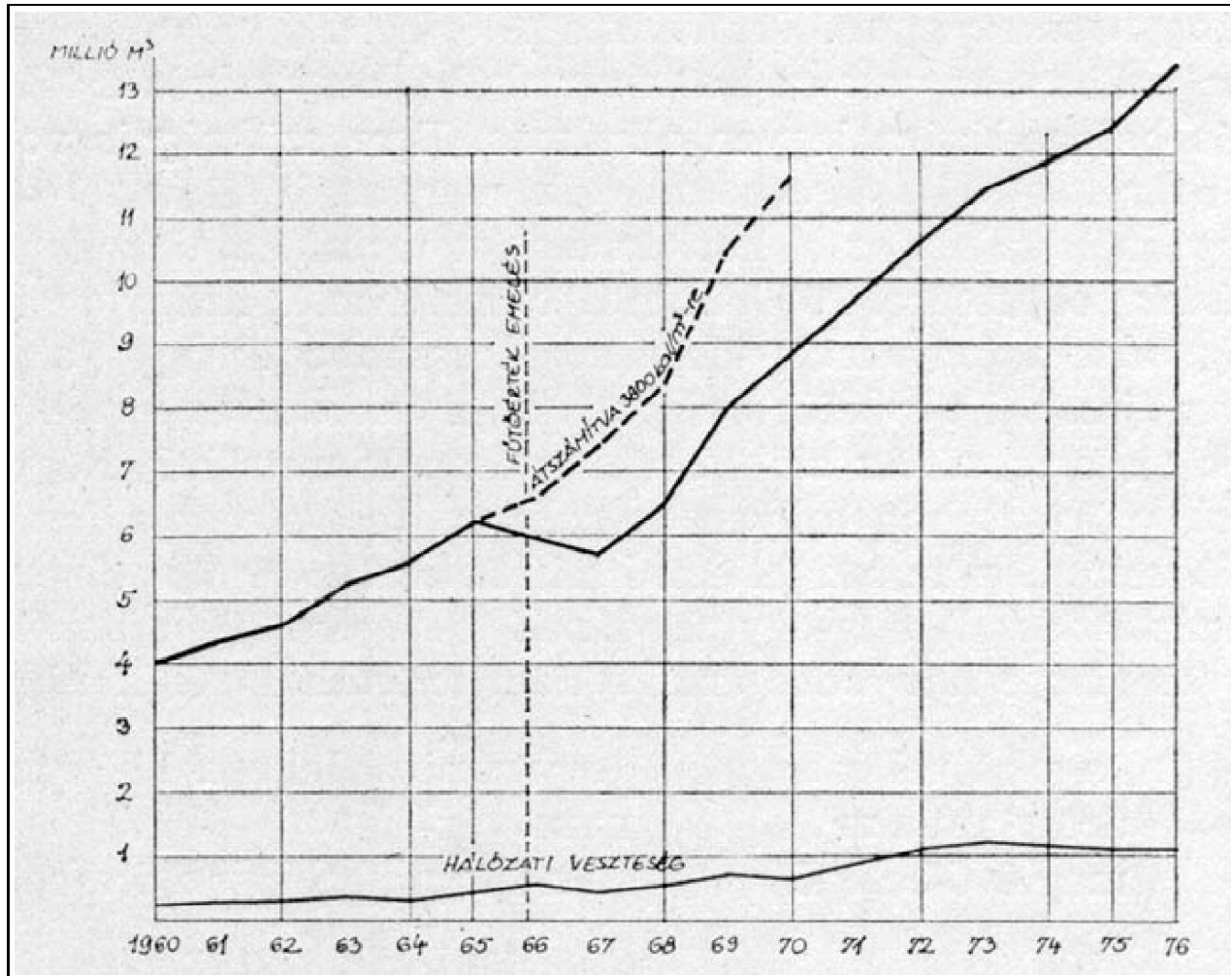
21. A gáztermelés az 1960–1976. években
