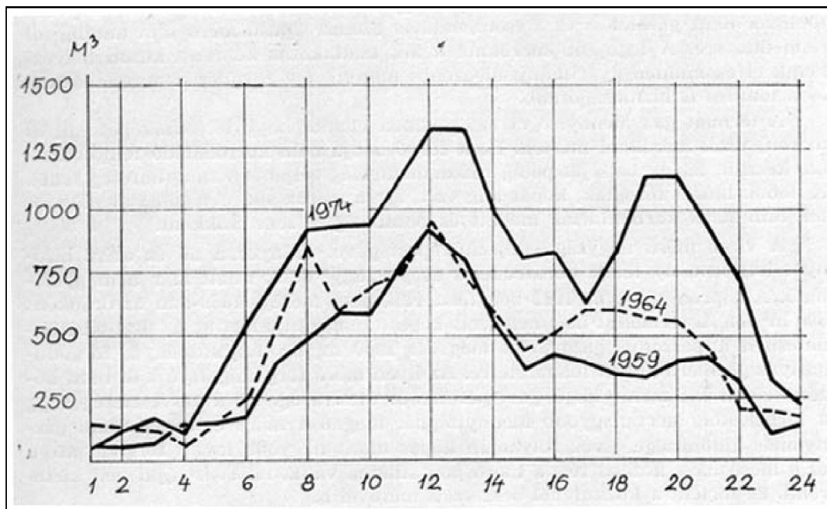
32/b. Óránkénti gázleadás egy-egy júliusi hétköznapon (1959, 1964, 1974)
