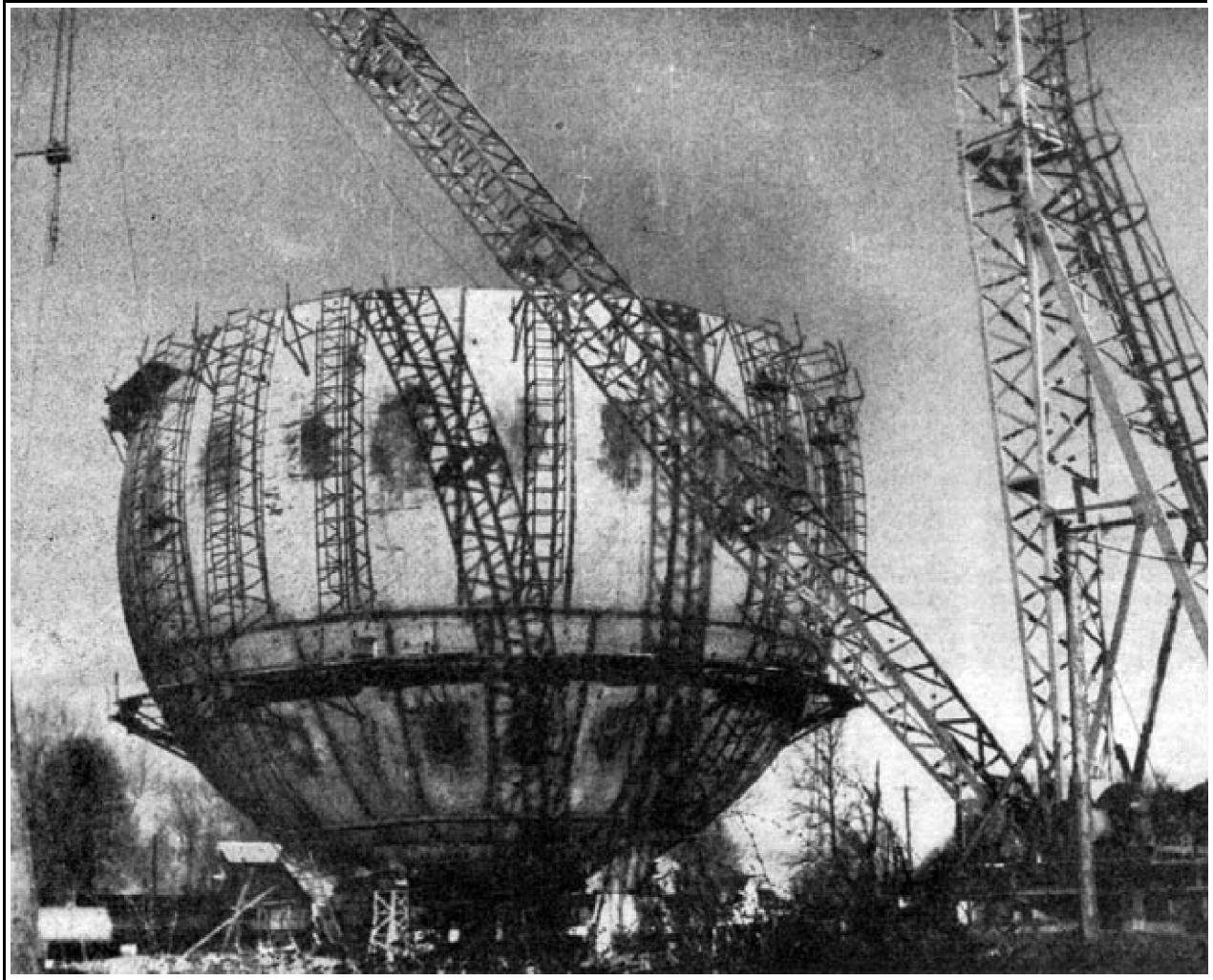
19. A gömbgáztartó szerelése (1965)
