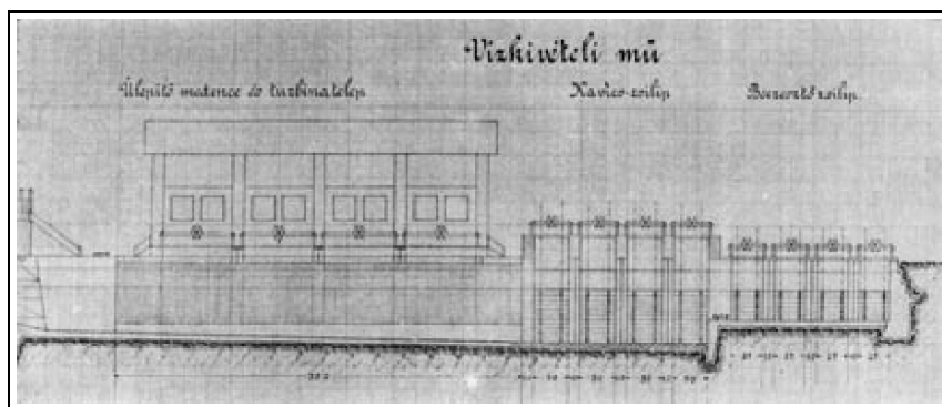
1213. A nicki víztelep terve (1920)
