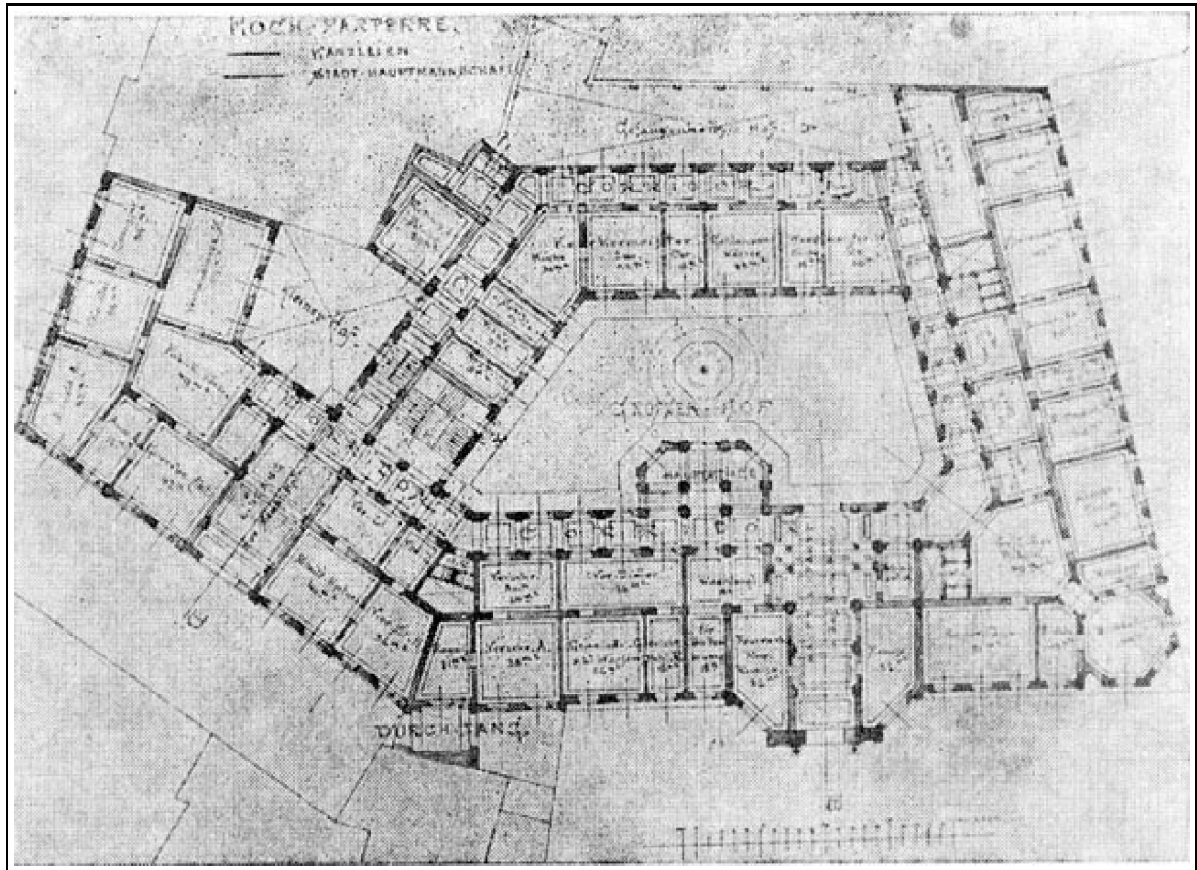
30423. Schachner Frigyes terve (homlokzat, földszint)
