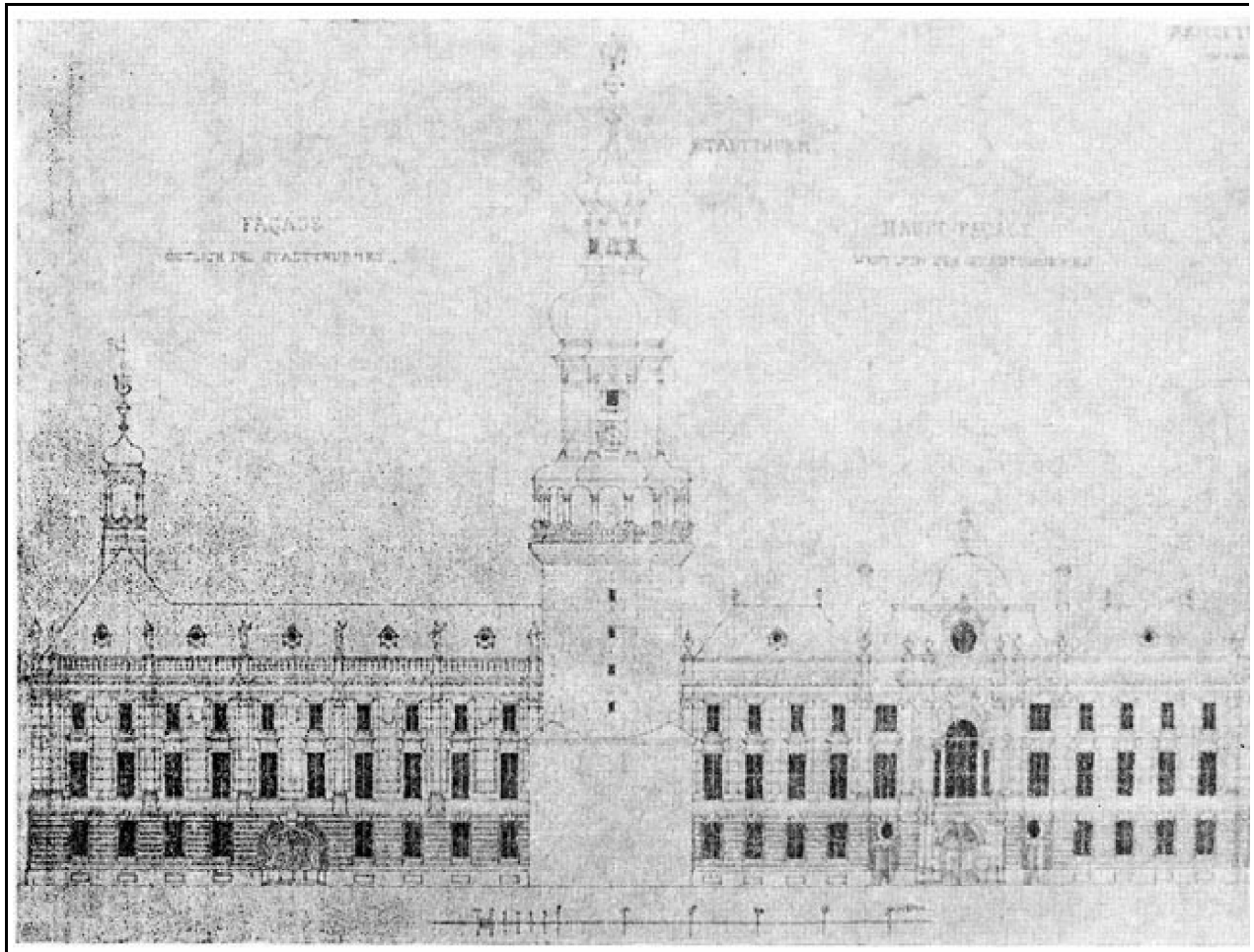
22. Schachner Frigyes terve (homlokzat)
