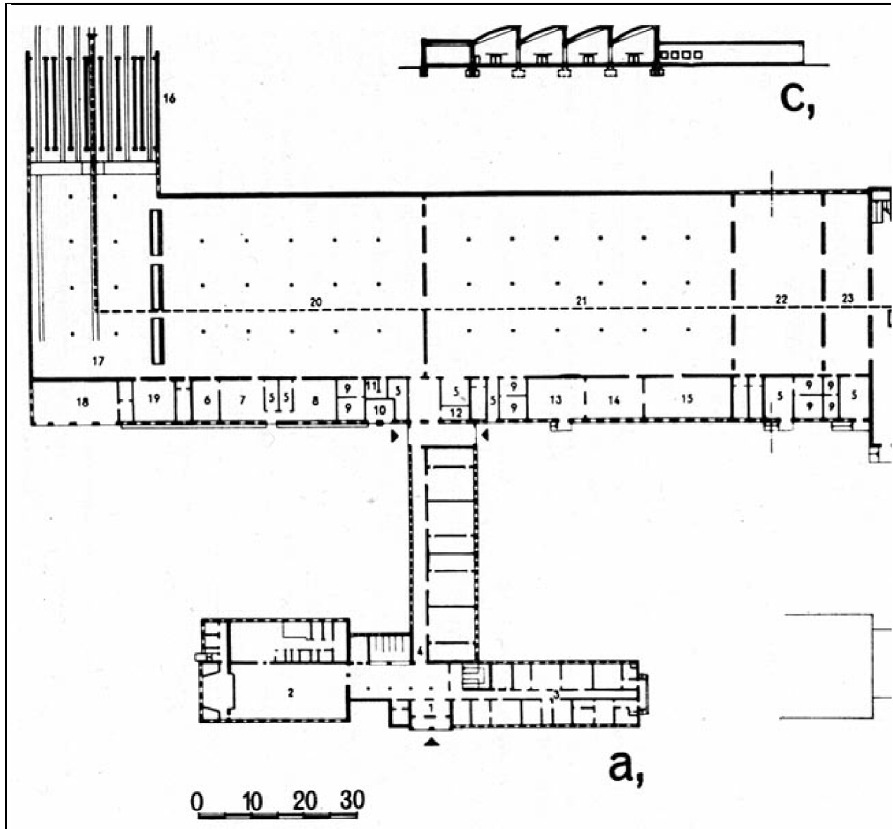
2073. Alaprajzok és az üzemi épület keresztmetszete a gépi műhelyen át.
