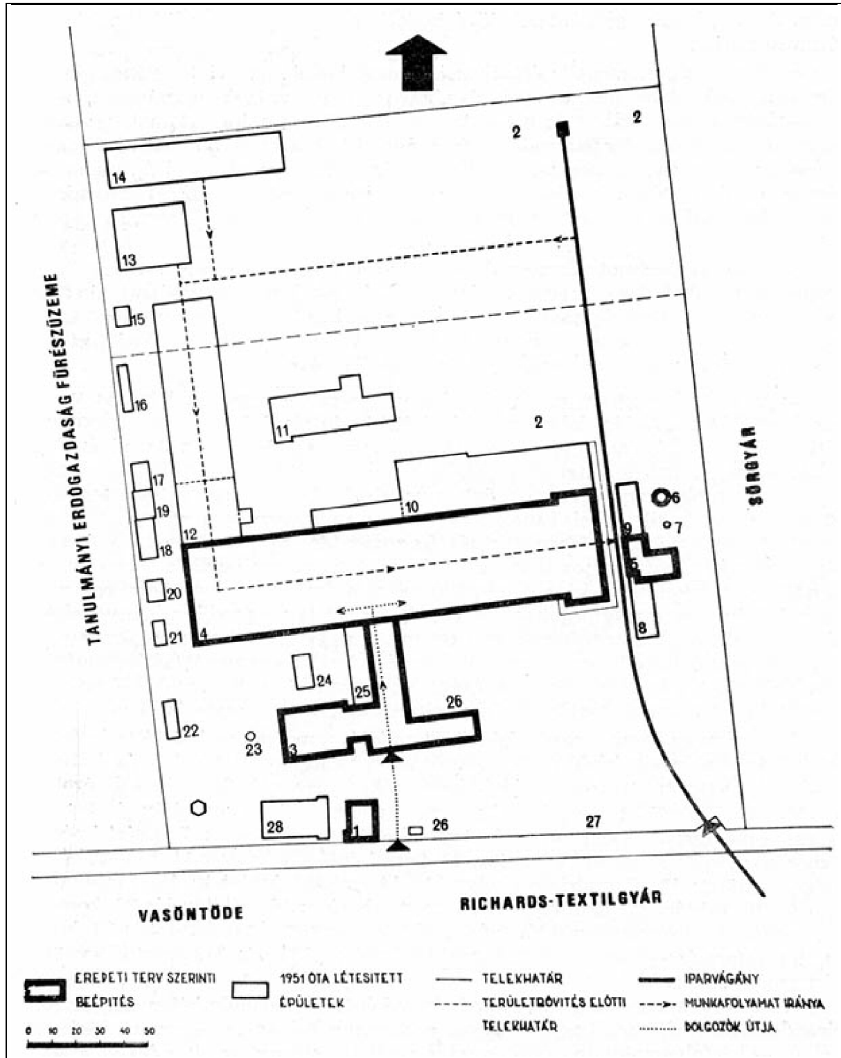
2041. A Soproni Épületasztalosárugár elrendezési rajza
