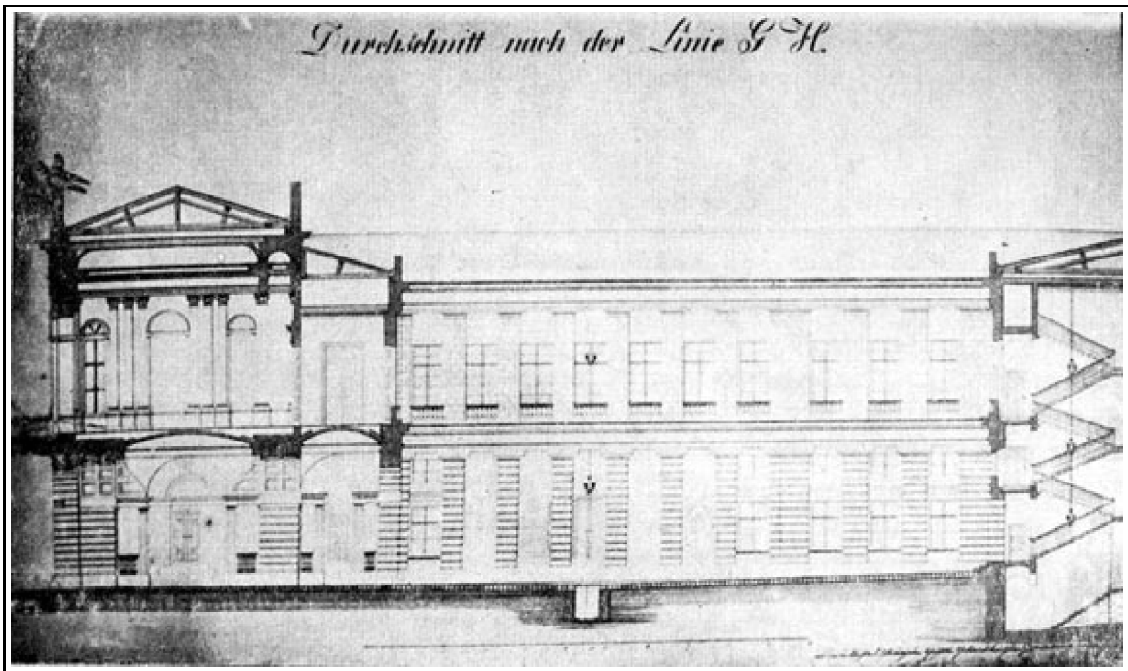
18. Stampf Ferenc harmadik terve. Oldalhomlokzat és metszet
