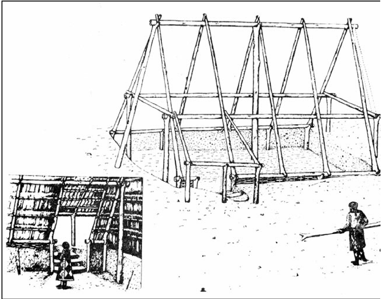
1544. A 9. sz. ház második építési periódusa cölöprendszerének rekonstrukciója
