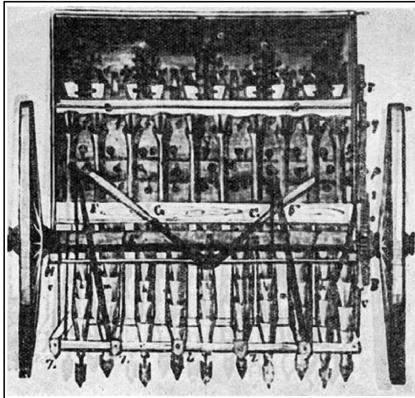
A Garret vetőgép. A Mezei Gazdaság Könyve, III. kötet, 283. kép
