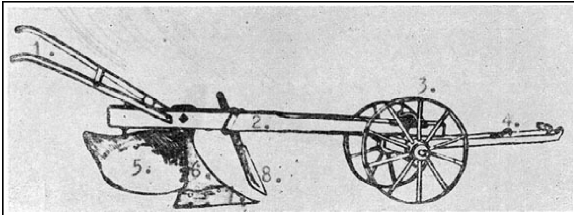
Vasfejű eke. (A magyarság néprajza, II. kötet 623. kép) 1. Ekeszarv. 2. Gerendely. 3. Taliga. 4. Taligarúd. 5. Kormány. 6. Ekefej. 7. Laposvas vagy ekevas. 8. Csoroszlya vagy hosszúvas
