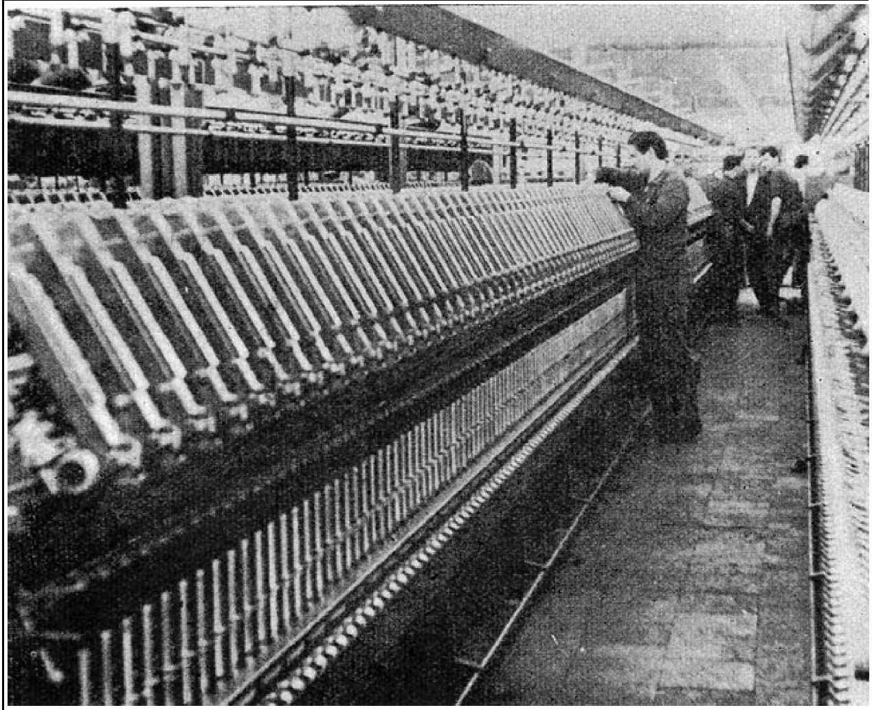
Richards Fésűsfonó. Olasz automata gépsor beállítása
