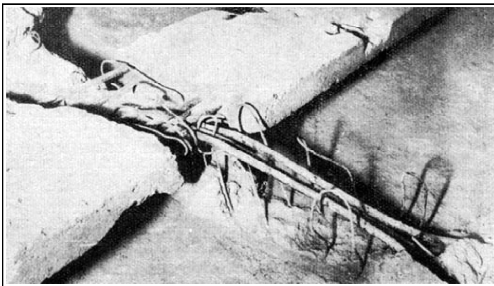
A vasbeton erkélyszerkezet szabaddá vált vasbetétei
