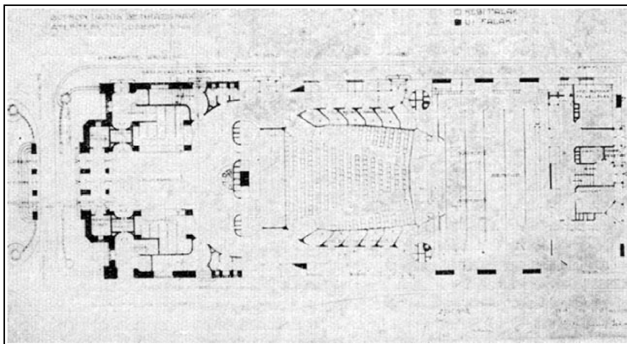
A színház tervének földszinti alaprajza
