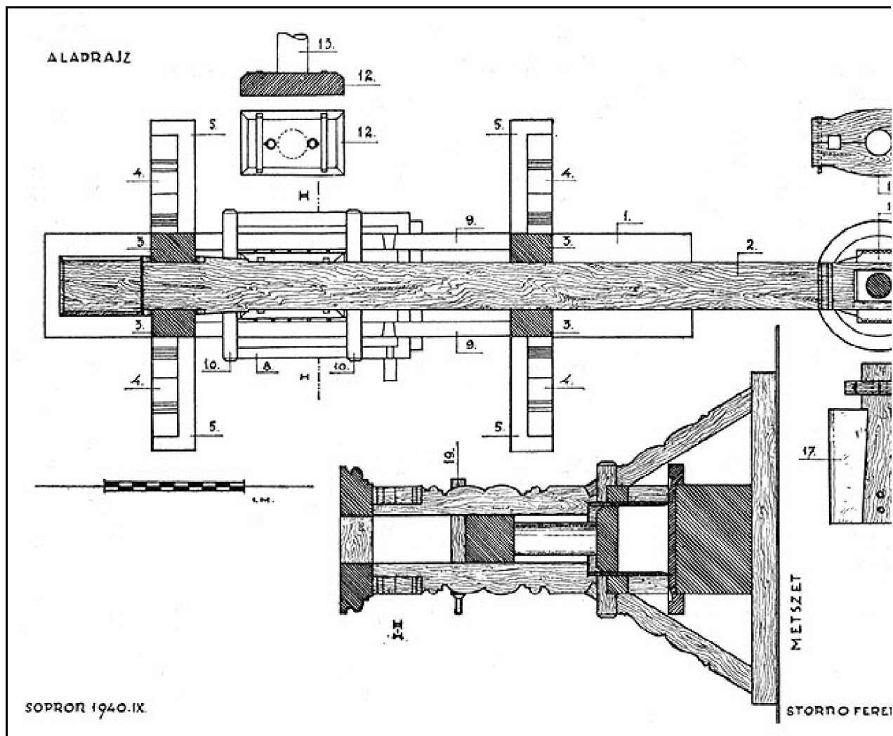
2. kép. Borsajtó a Storno-házban. (Alaprajz és metszet.)
