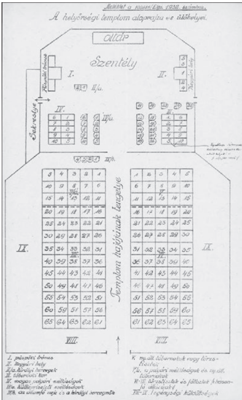
A budavári helyőrségi templom alaprajza és ülőhelyei, 1932
