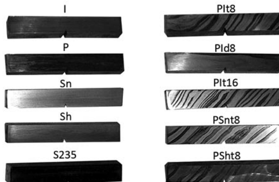
3. ábra: Bucavashól kovácsolt Charpy próbatestek (reprezentáns darab egy-egy próbatest típusból) A felület polírozva és 2%-os nitállal maratva
